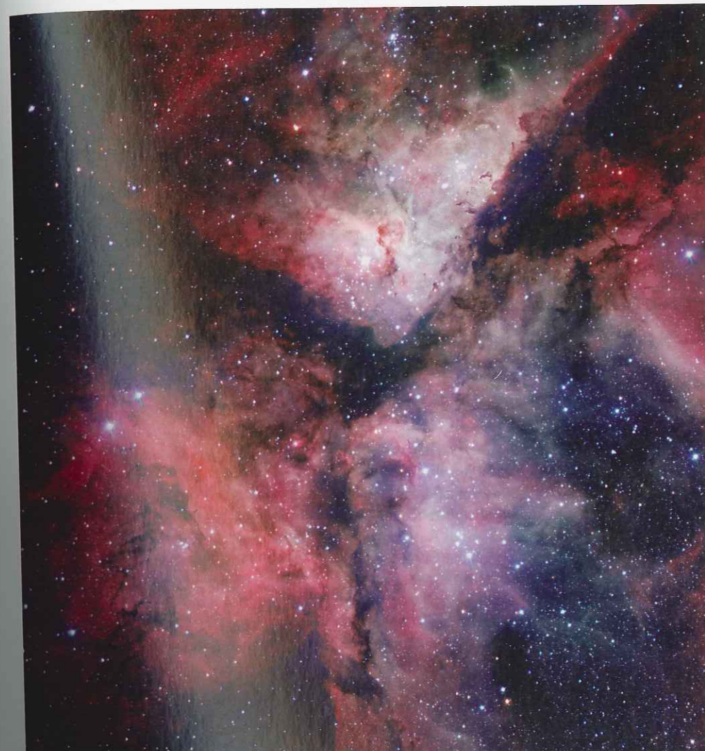
Carina nebula, la Nebulosa della Carena, in una immagine ripresa con il telescopio VST (Eso, Osservatorio australe europeo)
