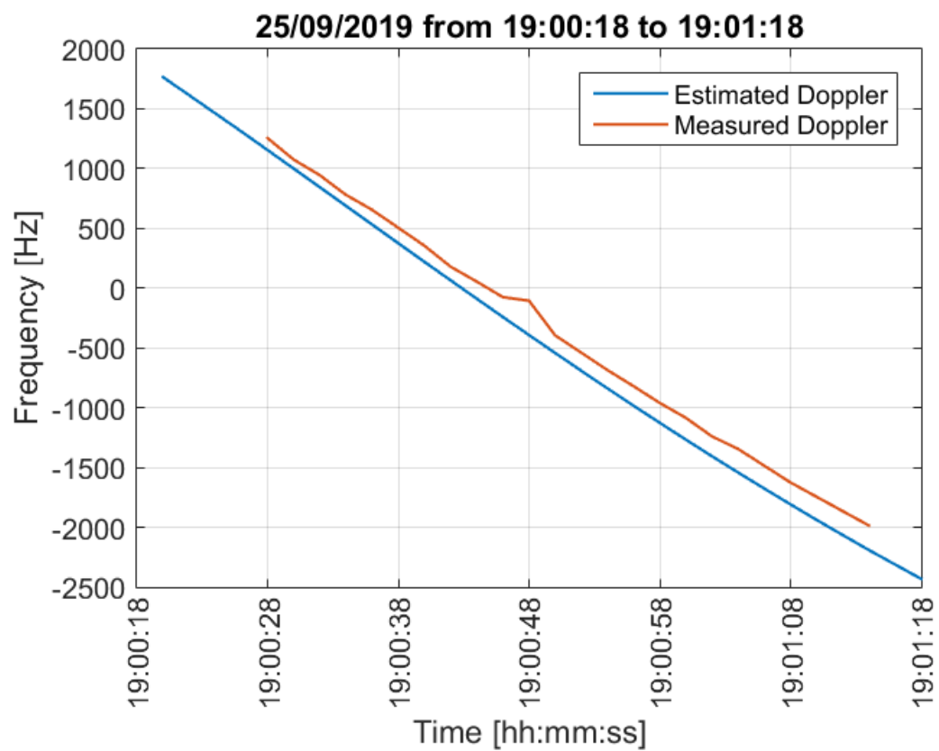
Figura 12. Confronto fra Doppler stimato e Doppler misurato su tutto il tempo di acquisizione per la misura del 25/09/2019.
