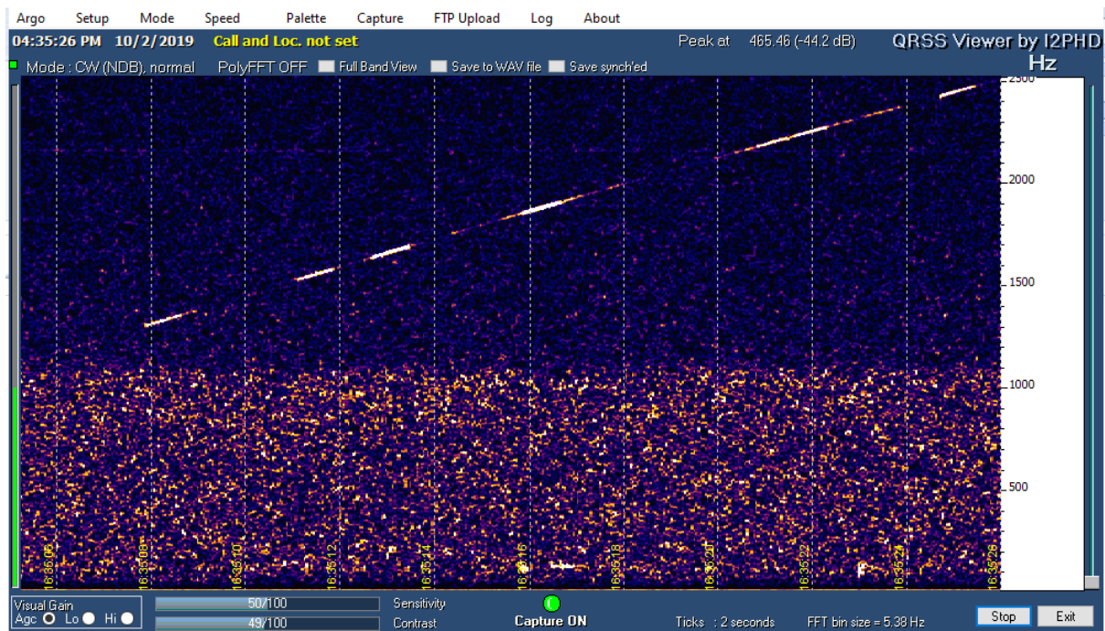
Figura 17. Schermate di acquisizione dell'eco Doppler della ISS nella giornata 02/10/2019: a) dalle 16:34:34 alle 16:34:52, b) dalle 16:34:52 alle 16:35:08, c) dalle 16:35:08 alle 16:35:26.
