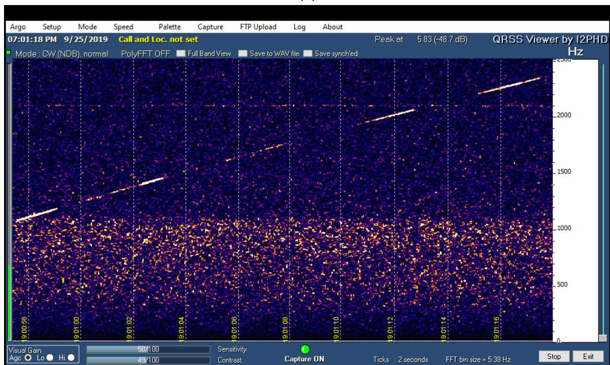
Figura 11. Schermate di acquisizione dell'eco Doppler della ISS nella giornata 25/09/2019: a) dalle 19:00:26 alle 19:00:44, b) dalle 19:00:44 alle 19:01:00, c) dalle 19:01:00 alle 19:01:17.
