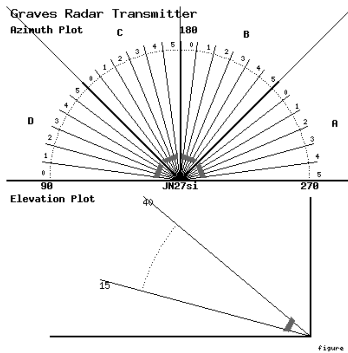
Figure 1. Rappresentazione del fascio del GRAVES in Azimut e Elevazione.
