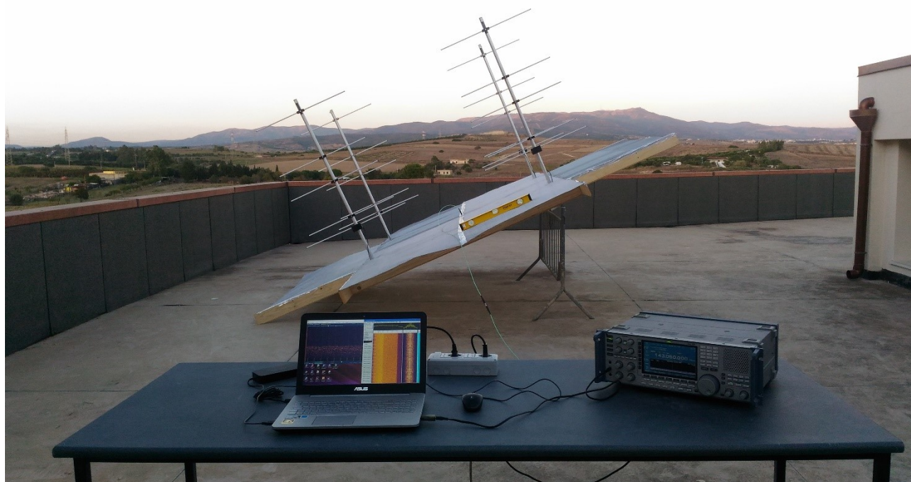
Figura 4. Foto del sistema ricevente costituito dall'array di YAGI.
