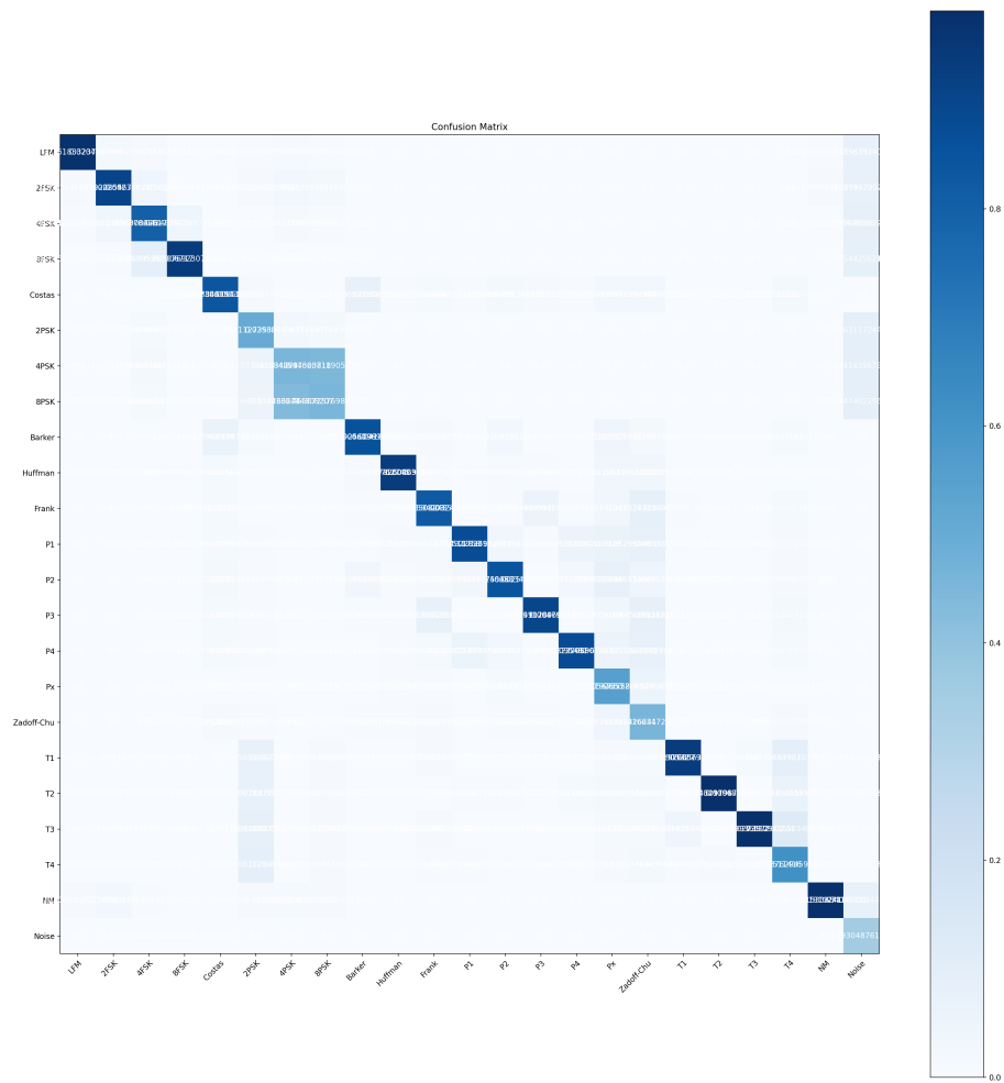
Figura 4.3: Confusion Matrix con addestramento di parte del dataset (SNR da 0 a 20 con passo di 2)
