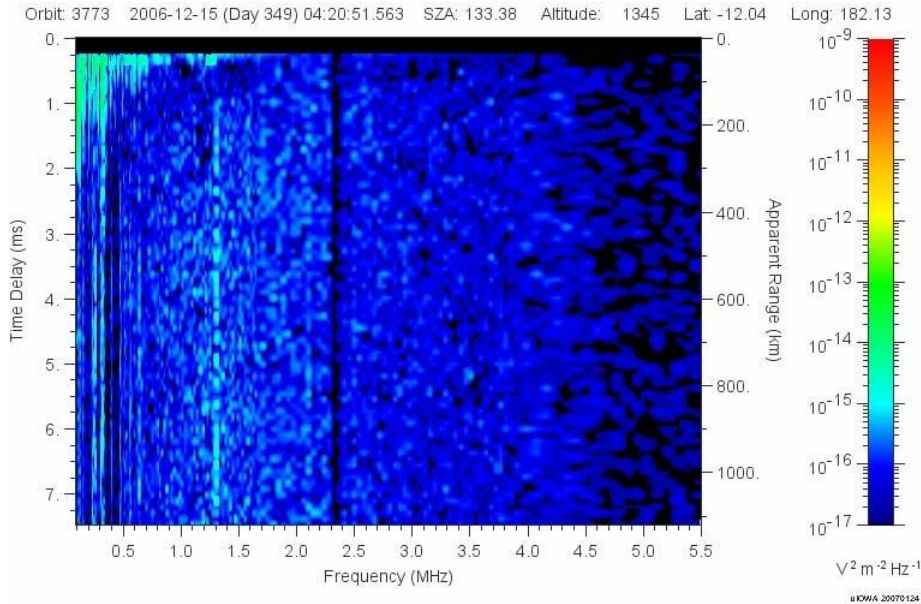
Fig. 4.1.1 (MARSIS AIS Ionogram, Orbit 3773)
