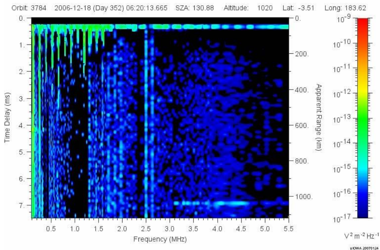
Fig. 4.3.1 (MARSIS AIS Ionogram, Orbit 3784)
