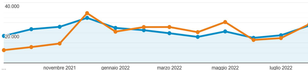
Figura 3: andamento dei visitatori mensili medi di EduINAF nel 2021/2022 (in blu) a confronto con i lettori medi dell'anno precedente (in arancione). (Fonte: Google Analytics)
