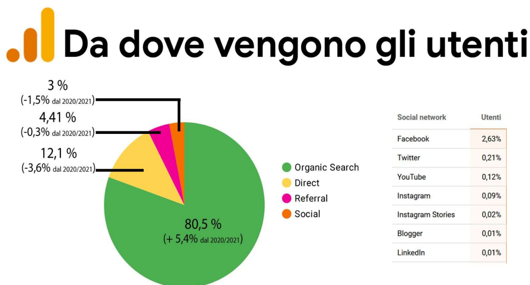
Figura 4: percentuale di lettori arrivata su EduINAF nel periodo in considerazione, in funzione dei canali di acquisizione. I dati sono confrontati con i valori dell'anno precedente. (Fonte: Google Analytics)
