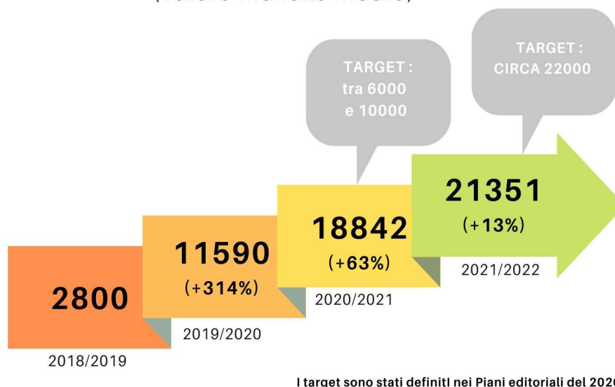
Figura 1: andamento dei visitatori mensili medi di EduINAF. (Fonte: Google Analytics)
