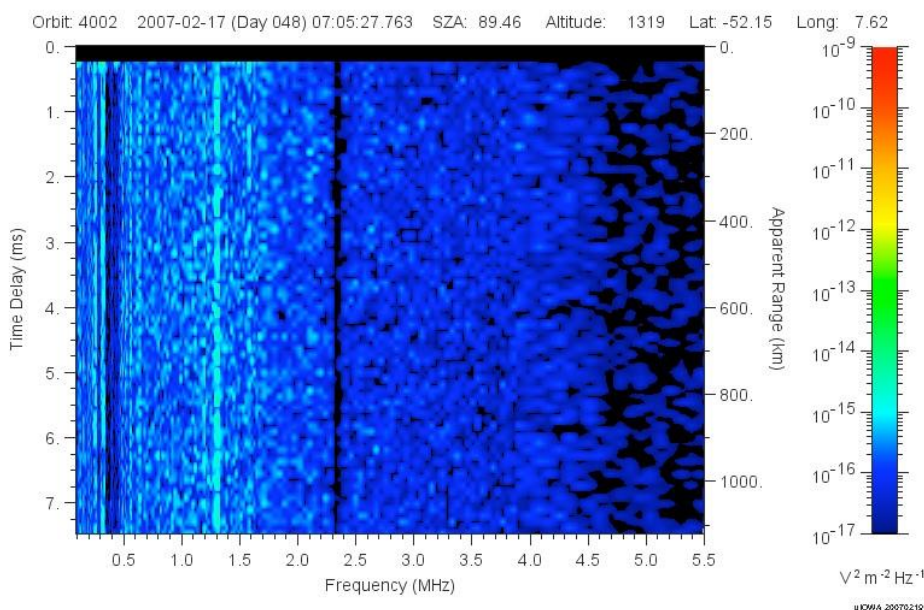
Fig. 4.1.1 (MARSIS AIS Ionogram, Orbit 4002)
