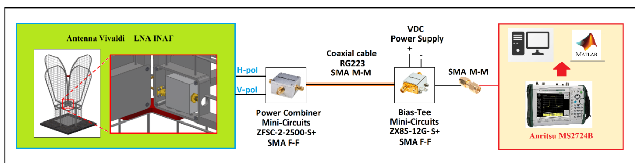
Figura 1 – Schema della catena di componenti a microonde per l'acquisizione del segnale usata per la campagna di misure RFI. La catena è composta da un LNA per ciascun canale di polarizzazione dell'antenna Vivaldi, da un power combiner che combina i due canali di polarizzazione, da un Bias-Tee utile per l'alimentazione degli LNA e da un analizzatore di spettro usato come back-end [6].
