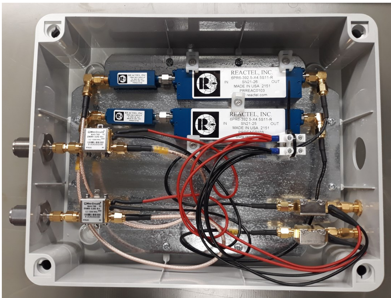
Figura 5 – (a) schema dei componenti a radio frequenza installati all'interno della scatola di derivazione; (b) foto della scatola di derivazione.
