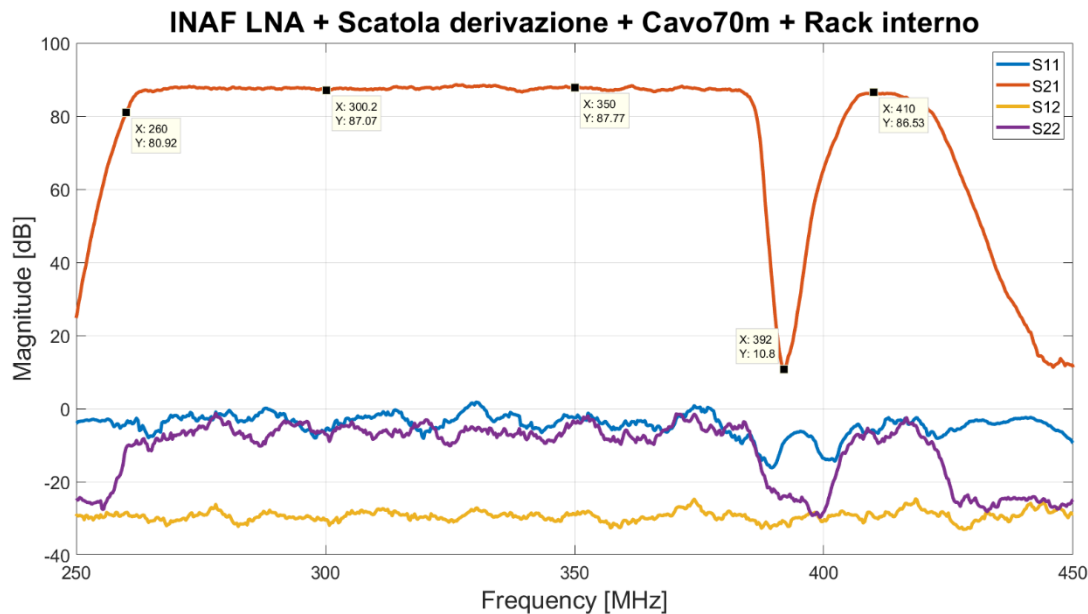
Figura 14 – Parametri S dell’intera catena ricevente del sistema SADino , precursore dell’array SAAD.
