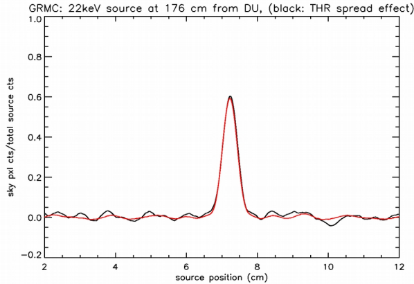
figura 4 Montecarlo: confronto tra l'immagine prodotta su un rivelatore con strip omogenee in soglia (curva rossa) e strip con la distribuzione di soglia ottenuta dai run di soglia sulla DU #1 (curva nera)
