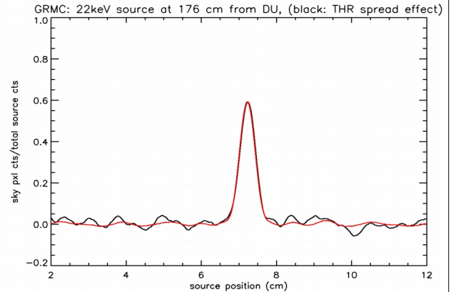
figura 5 Montecarlo: confronto tra l'immagine prodotta su un rivelatore con strip omogenee in soglia (curva rossa) e strip con la stessa distribuzione di soglia utilizzata per la figura precedente ma con un offset di 2.5 keV (curva nera).
