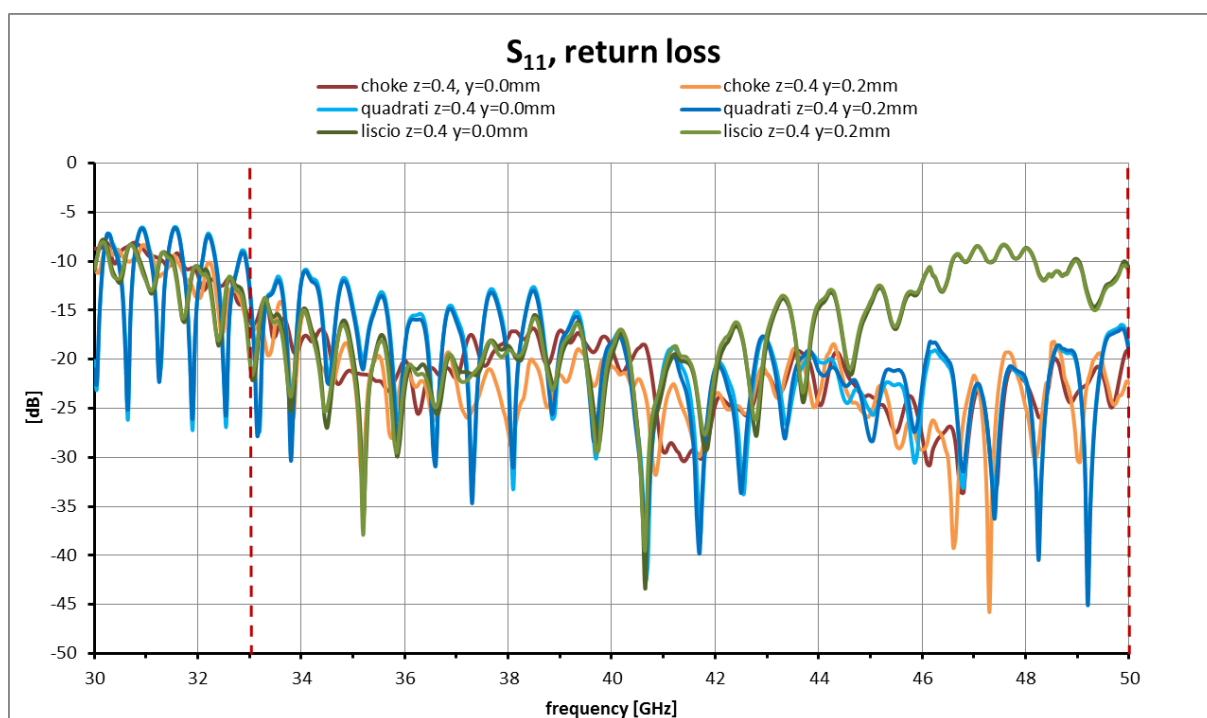
Fig. 5.3 Return loss dei tre tipi di gap termico
