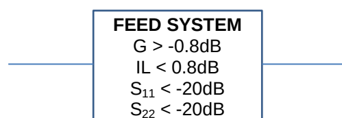
Fig. 2.10 Principali prestazioni del modulo Feed System
