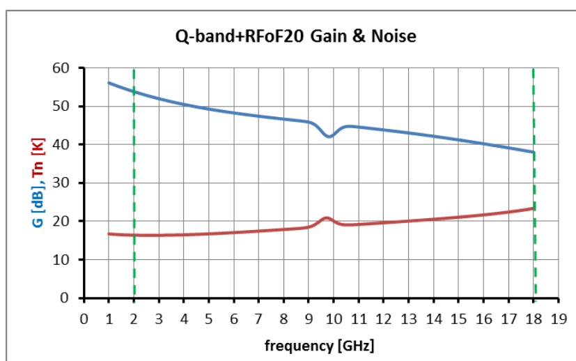
Fig. 8.1 G(f) e T_n(f) del ricevitore Qband + link ottico
