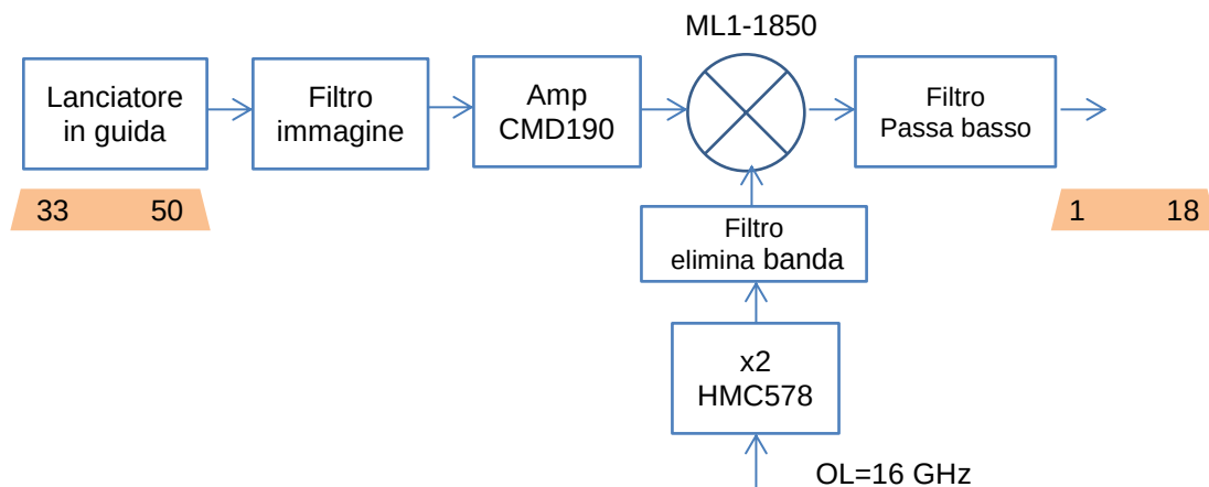
Fig. 4.2 Schema a blocchi modulo Qconv (1IF)
