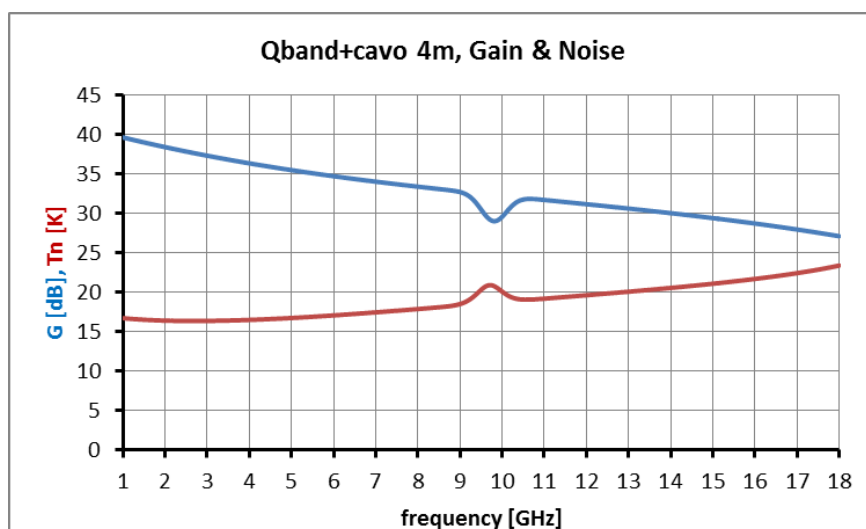
Fig. 8.5 G(f) e Tn(f) ricevitore Qband
