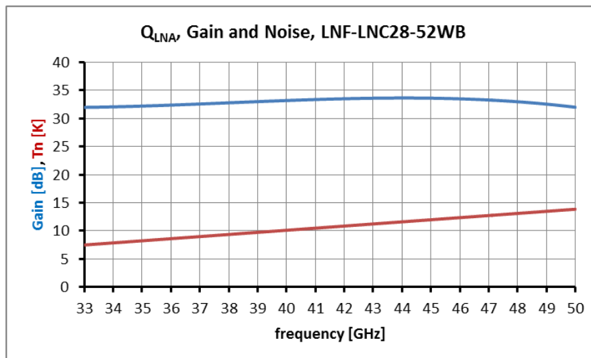
Fig. 3.2 Gain e Noise del LNA criogenico
