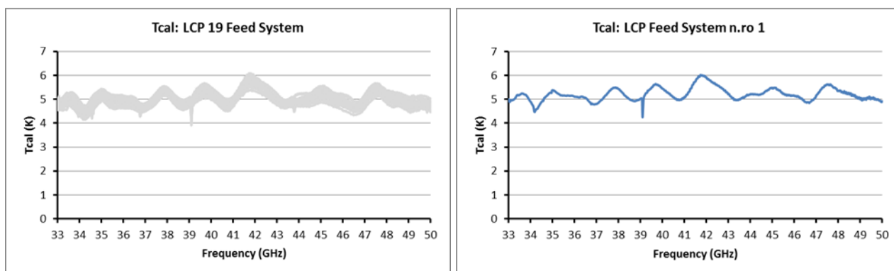
Fig. 10.7 19 feed system, a sinistra. Feed system n.ro 1 a destra. LCP. Equalizzazione con attenuatore.
