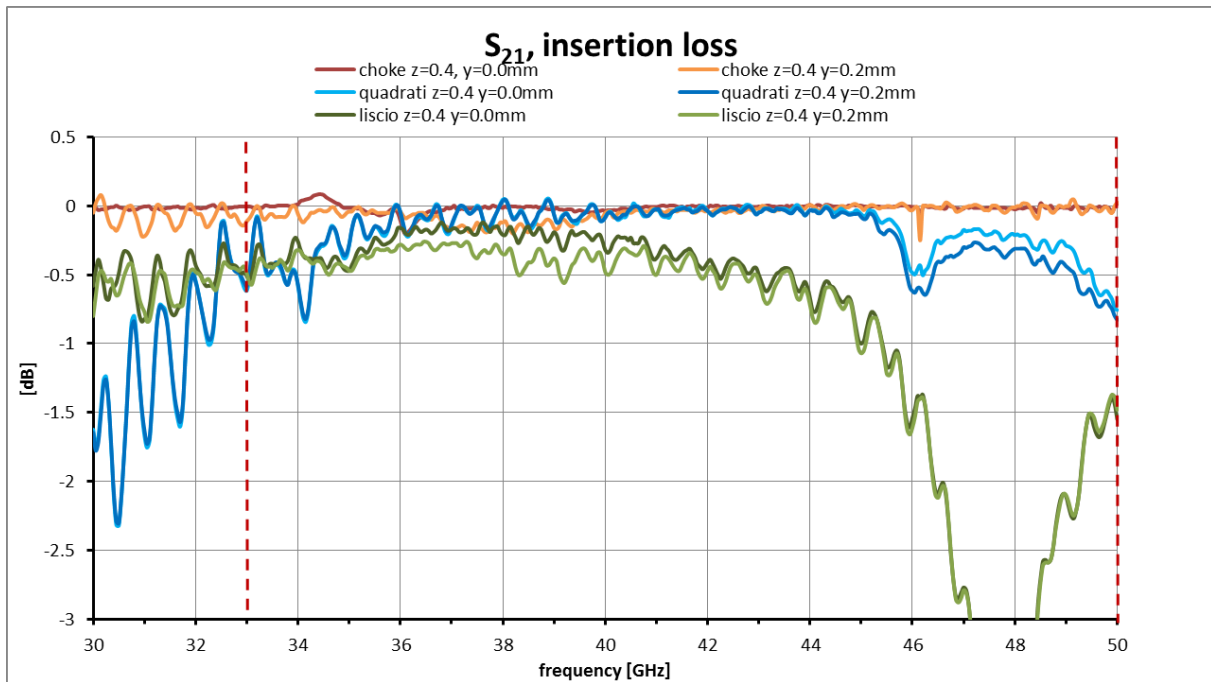
Fig. 5.4 Insertion loss dei tre tipi di gap termico
