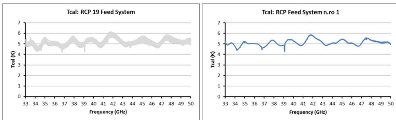
Fig. 10.8 19 feed system, a sinistra. Feed system n.ro 1 a destra. RCP. Equalizzazione con attenuatore.
