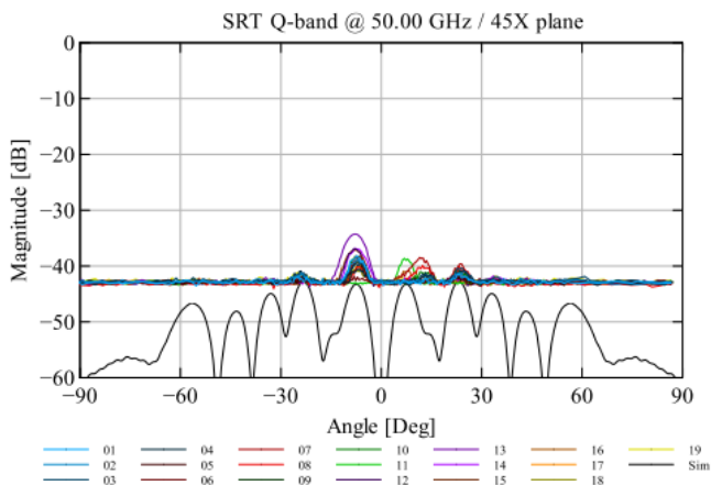
Fig. 2.3c 45°-plane 50GHz, 19 horn
