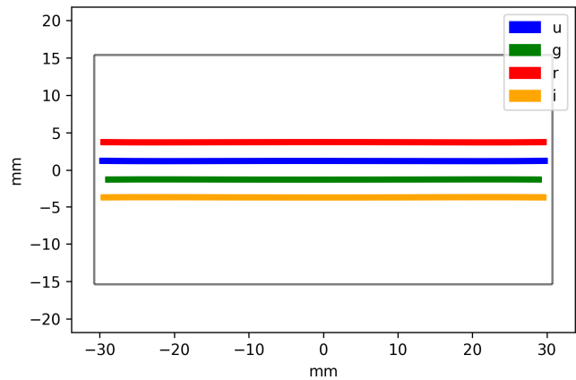
Figure 8. UV-VIS arm: spectral format.
