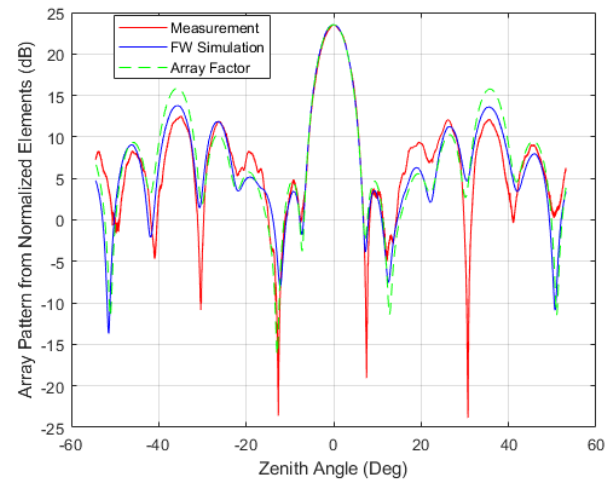
Fig. 4. preAAVS1 array (beam) patterns at 350 MHz.
