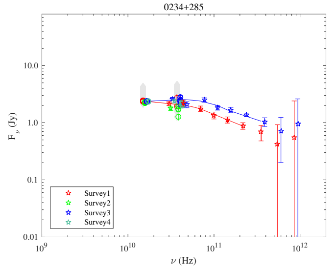
Fig. 1.12. 0234+285.
