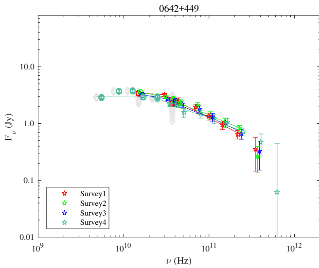
Fig. 1.29. 0642+449.
