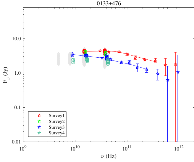
Fig. 1.7. 0133+476.
