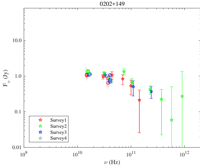
Fig. 1.9. 0202+149.
