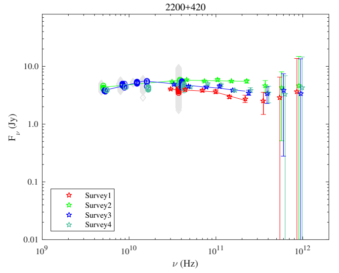
Fig. 1.94. 2200+420.
