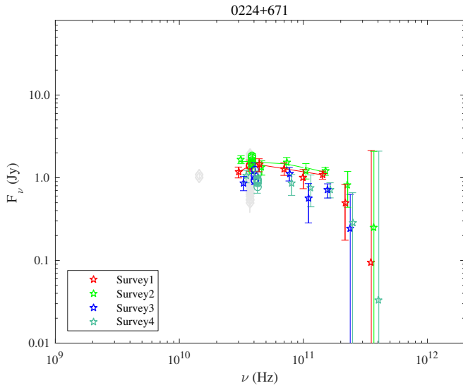
Fig. 1.11. 0224+671.
