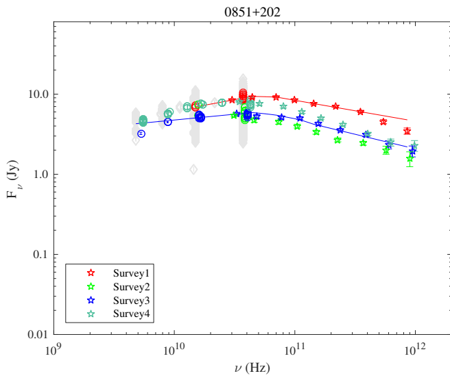
Fig. 1.41. 0851+202.
