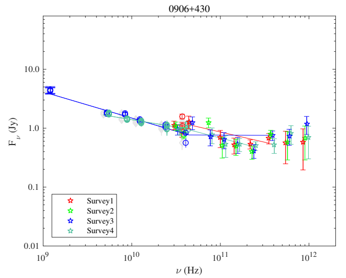
Fig. 1.42. 0906+430.
