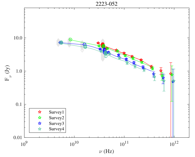
Fig. 1.98. 2223–052.
