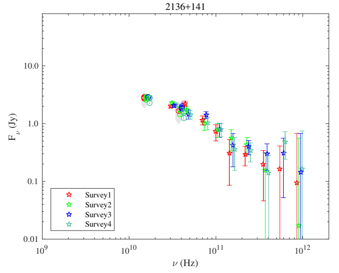
Fig. 1.92. 2136+141.
