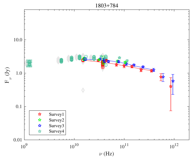
Fig. 1.78. 1803+784.
