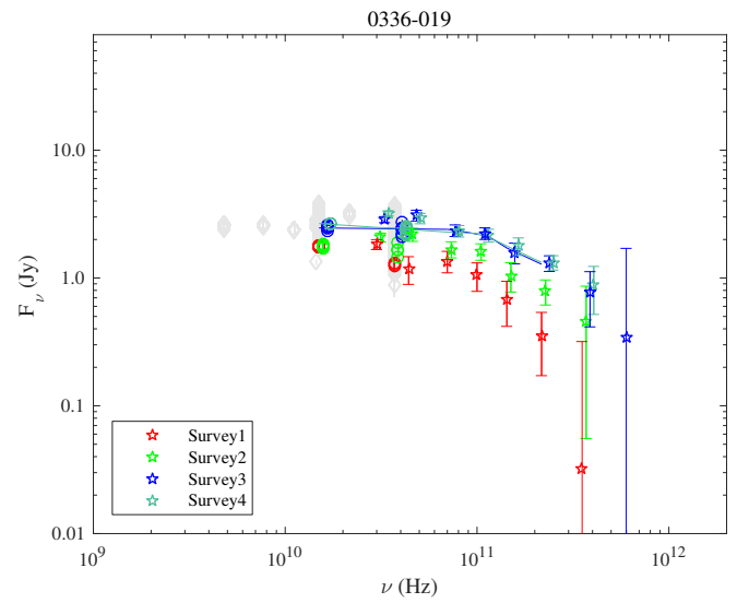
Fig. 1.18. 0336-019.
