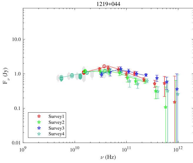
Fig. 1.55. 1219+044.
