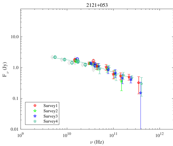
Fig. 1.89. 2121+053.
