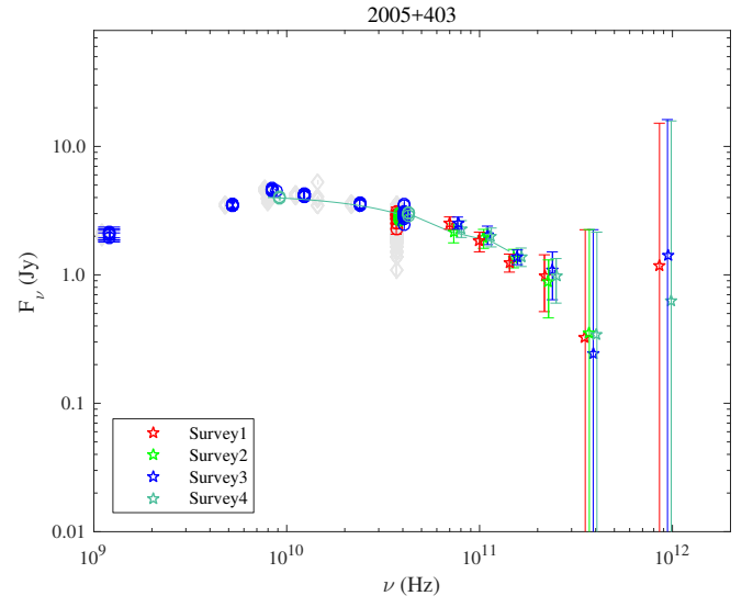
Fig. 1.86. 2005+403.
