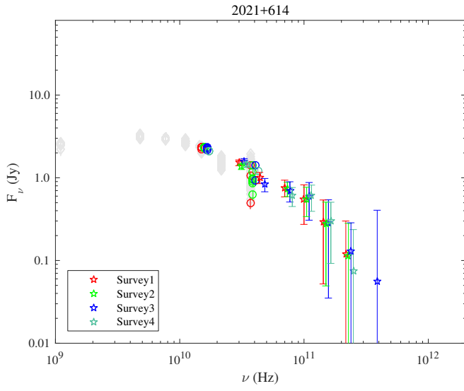
Fig. 1.87. 2021+614.
