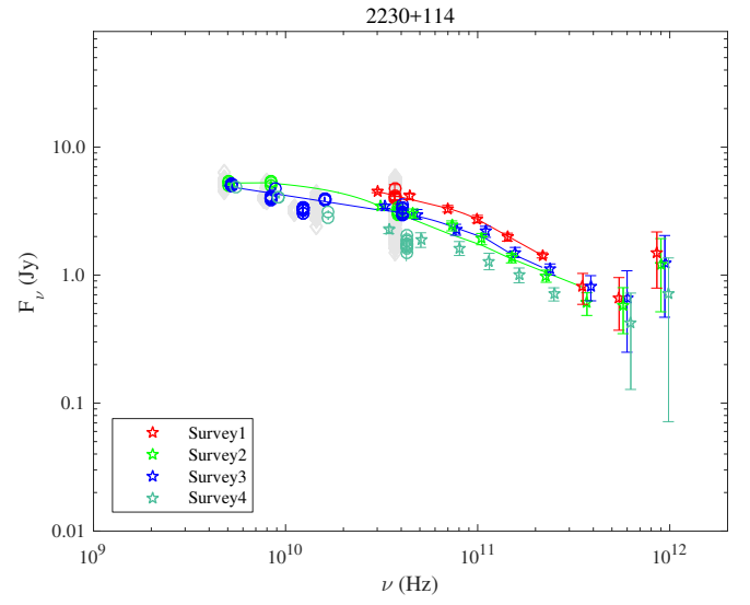
Fig. 1.100. 2230+114.
