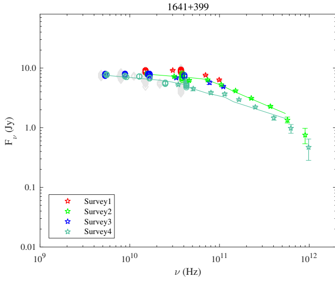
Fig. 1.73. 1641+399.
