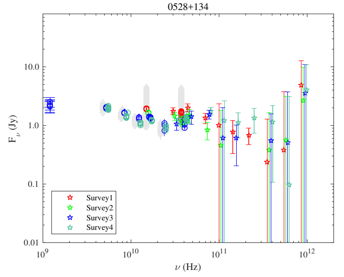
Fig. 1.26. 0528+134.
