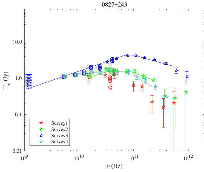
Fig. 1.39. 0827+243.
