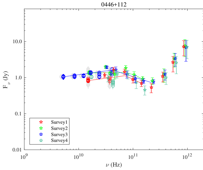
Fig. 1.23. 0446+112.
