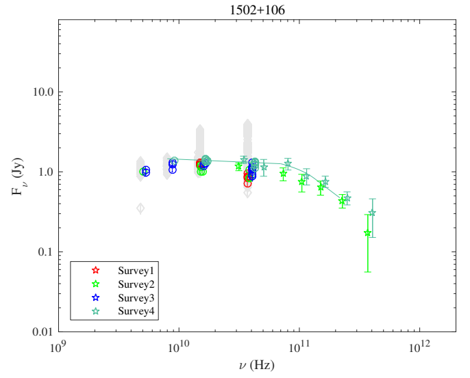
Fig. 1.64. 1502+106.
