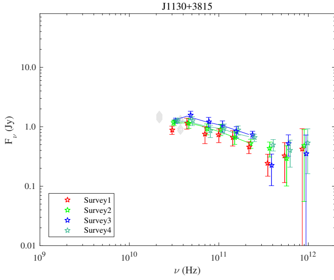
Fig. 1.51. J1130+3815.
