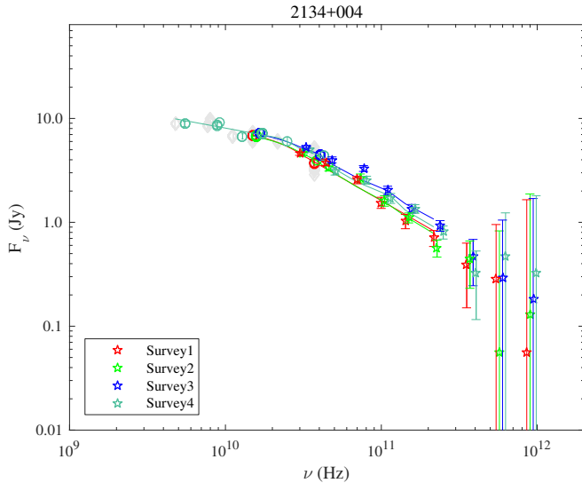
Fig. 1.91. 2134+004.
