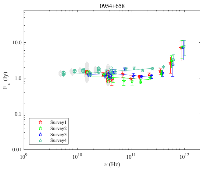
Fig. 1.47. 0954+658.
