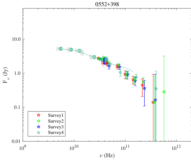
Fig. 1.27. 0552+398.
