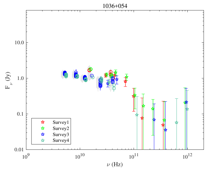
Fig. 1.48. 1036+054.
