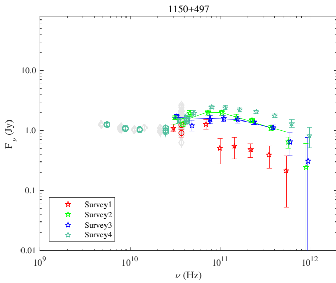
Fig. 1.53. 1150+497.
