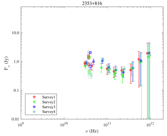
Fig. 1.104. 2353+816.
