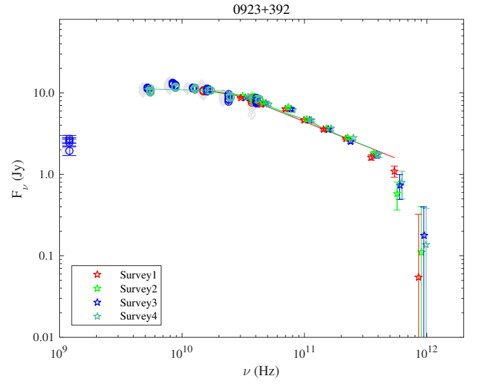
Fig. 1.44. 0923+392.
