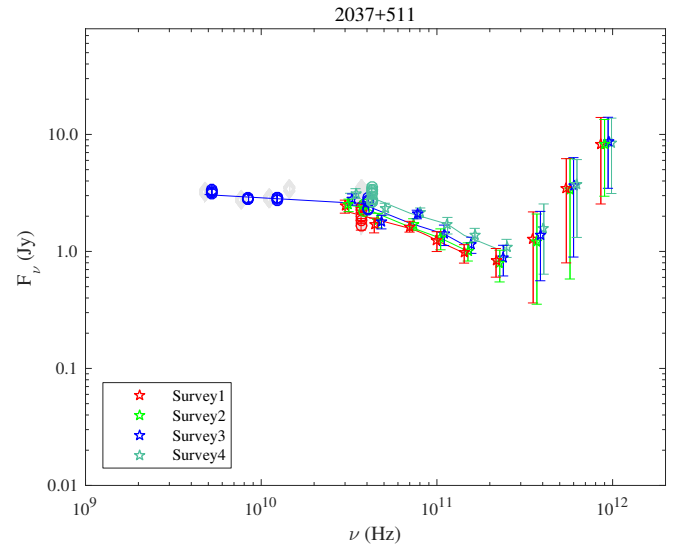
Fig. 1.88. 2037+511.
