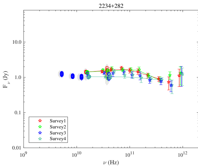
Fig. 1.101. 2234+282.
