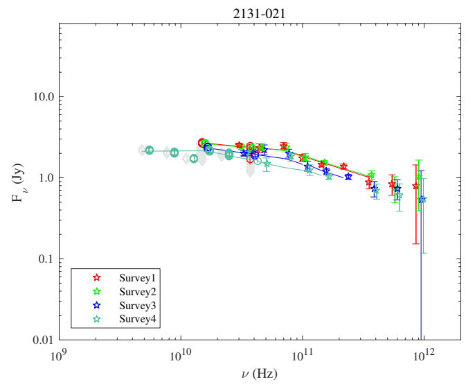
Fig. 1.90. 2131-021.
