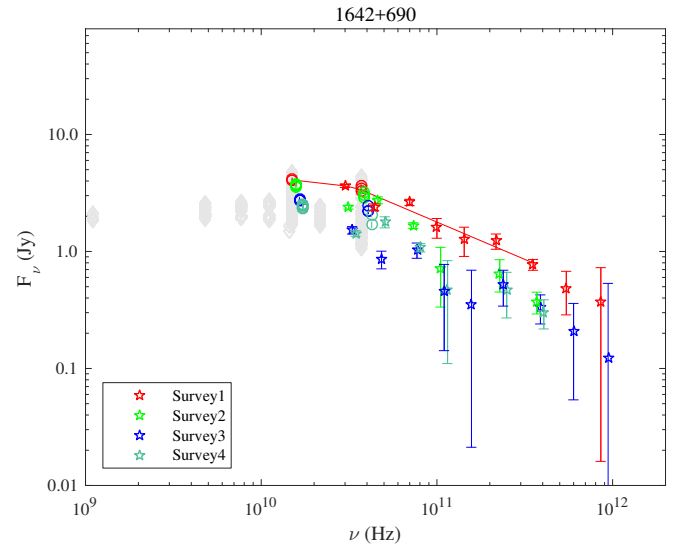
Fig. 1.72. 1642+690.
