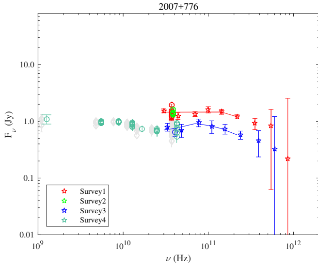
Fig. 1.85. 2007+776.
