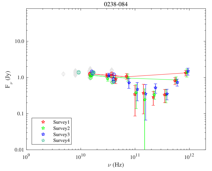
Fig. 1.14. 0238-084.
