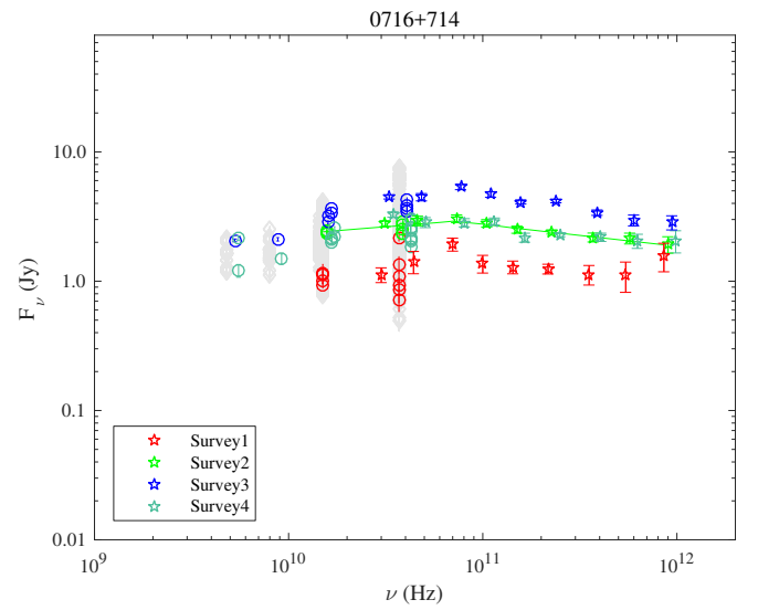
Fig. 1.30. 0716+714.
