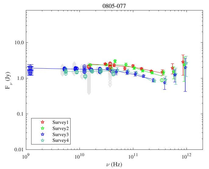
Fig. 1.36. 0805–077.
