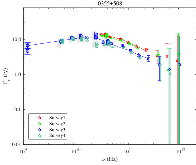
Fig. 1.19. 0355+508.
