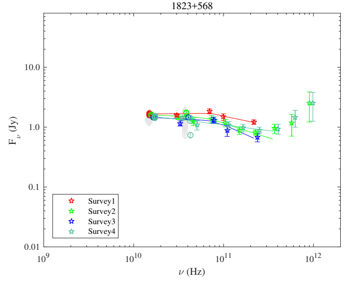
Fig. 1.80. 1823+568.
