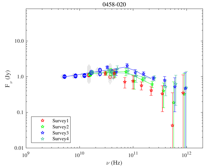
Fig. 1.24. 0458-020.
