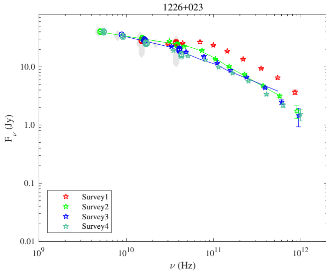
Fig. 1.57. 1226+023.
