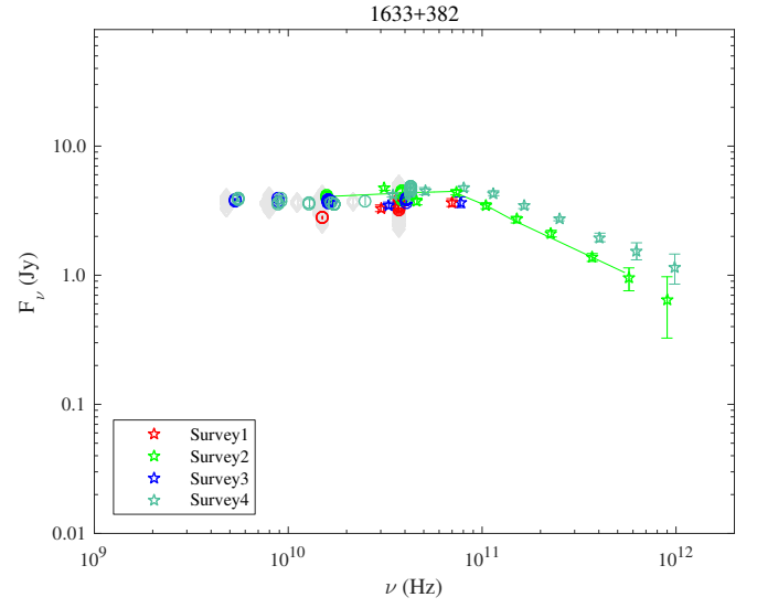
Fig. 1.70. 1633+382.
