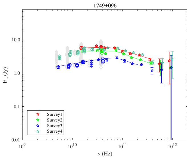
Fig. 1.77. 1749+096.
