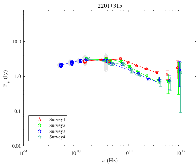
Fig. 1.95. 2201+315.
