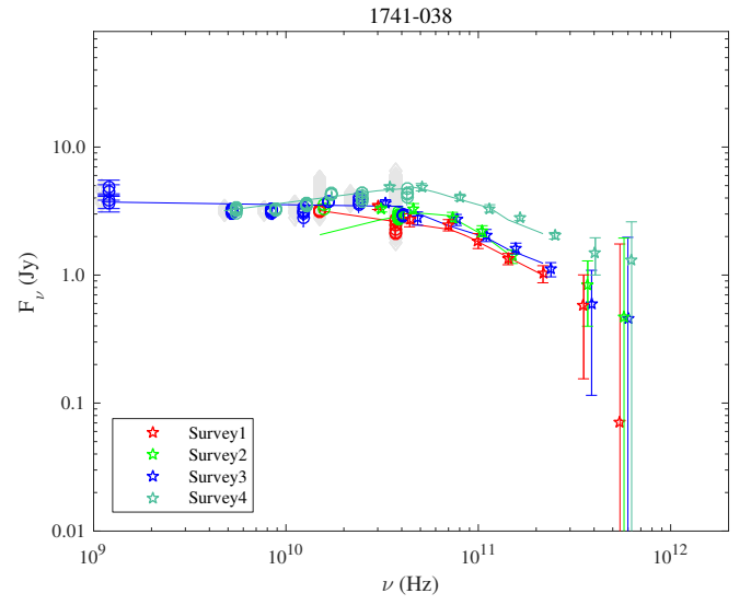
Fig. 1.76. 1741-038.
