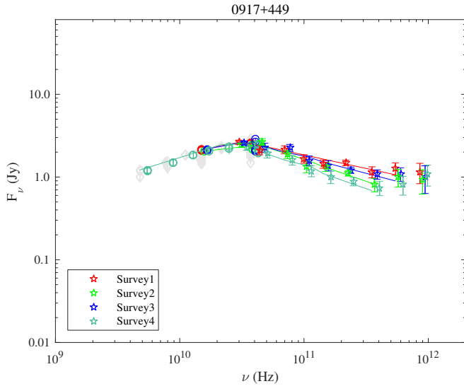
Fig. 1.43. 0917+449.
