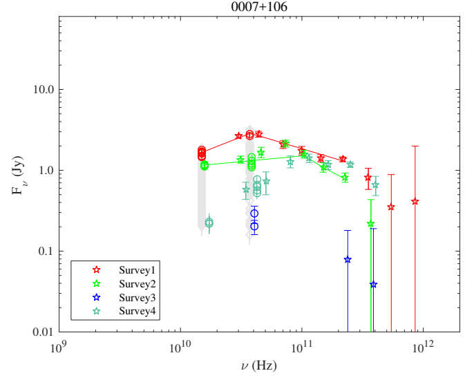
Fig. 1.2. 0007+106.
