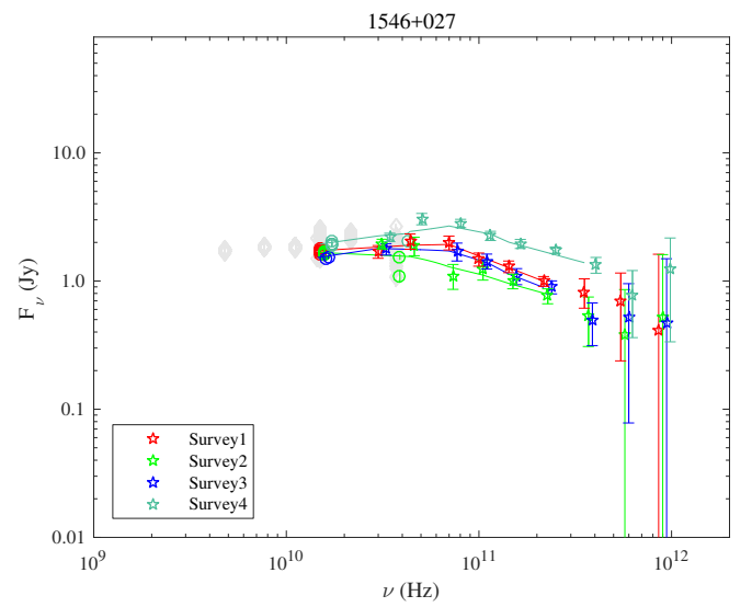
Fig. 1.66. 1546+027.
