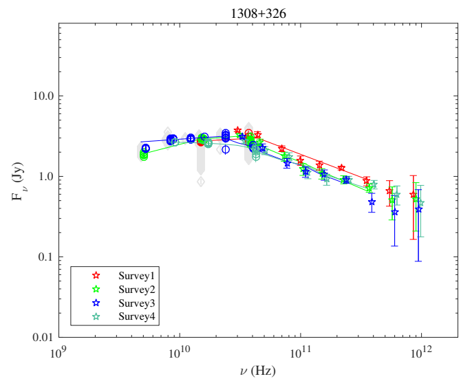
Fig. 1.60. 1308+326.
