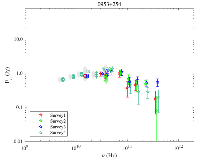
Fig. 1.46. 0953+254.
