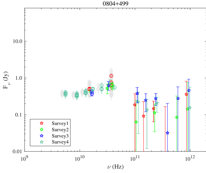
Fig. 1.37. 0804+499.
