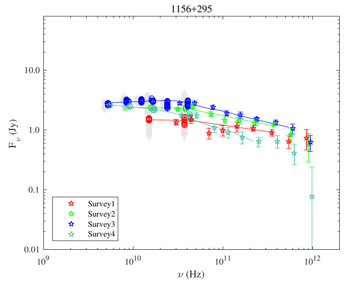
Fig. 1.54. 1156+295.
