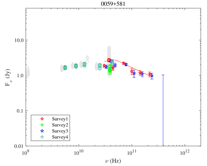
Fig. 1.4. 0059+581.
