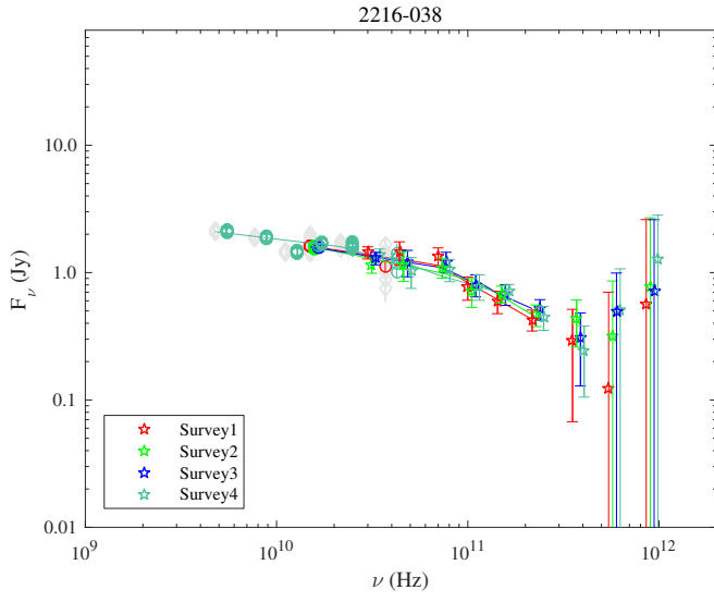
Fig. 1.97. 2216–038.
