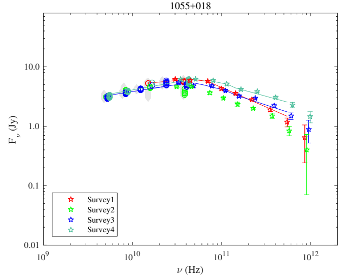
Fig. 1.50. 1055+018.
