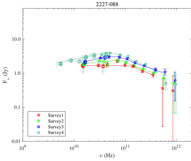
Fig. 1.99. 2227–088.
