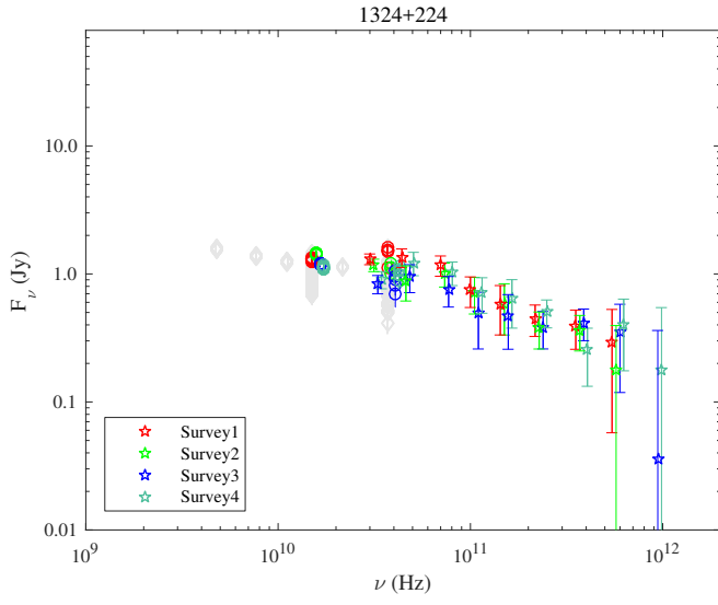
Fig. 1.61. 1324+224.
