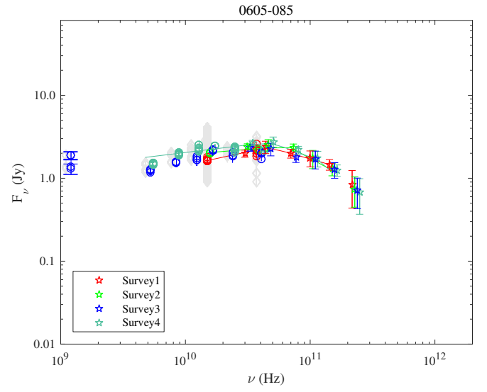
Fig. 1.28. 0605-085.
