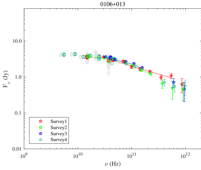
Fig. 1.5. 0106+013.
