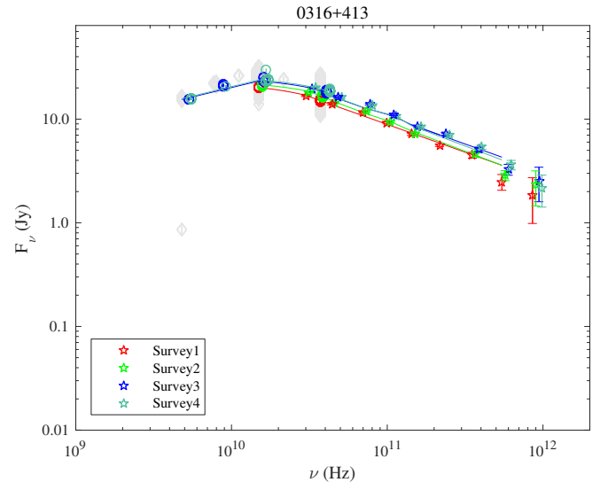
Fig. 1.16. 0316+413.
