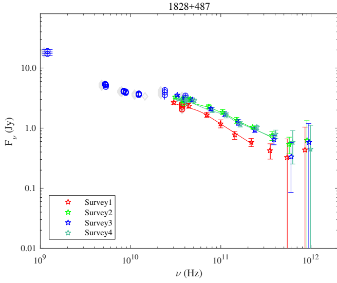
Fig. 1.81. 1828+487.
