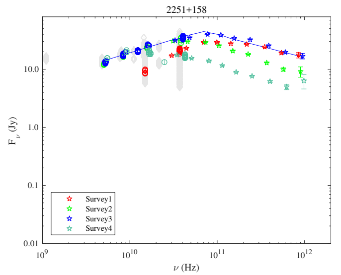
Fig. 1.102. 2251+158.
