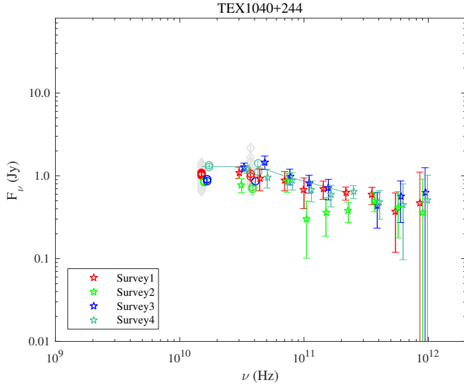
Fig. 1.49. TEX1040+244.
