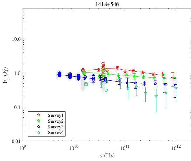
Fig. 1.63. 1418+546.
