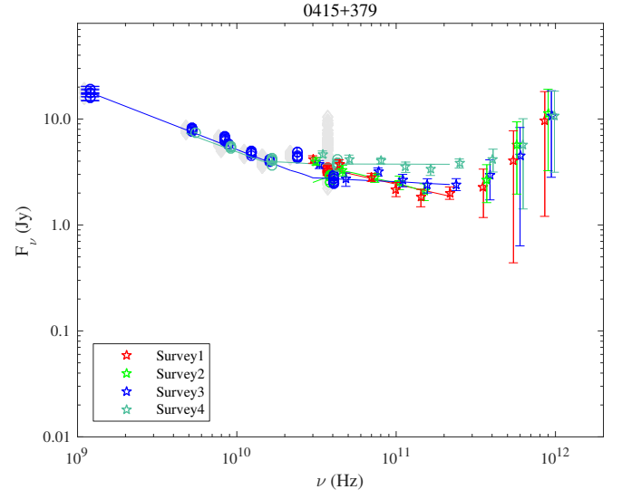
Fig. 1.20. 0415+379.
