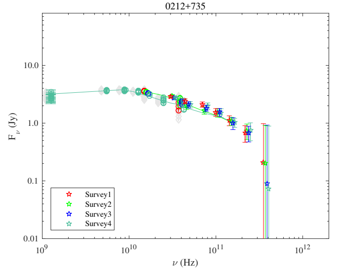
Fig. 1.10. 0212+735.
