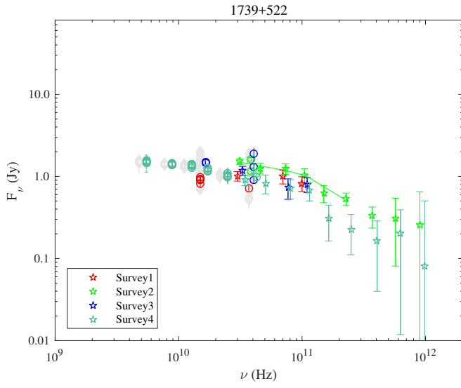
Fig. 1.75. 1739+522.
