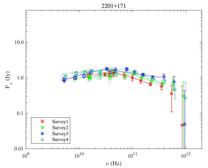
Fig. 1.96. 2201+171.
