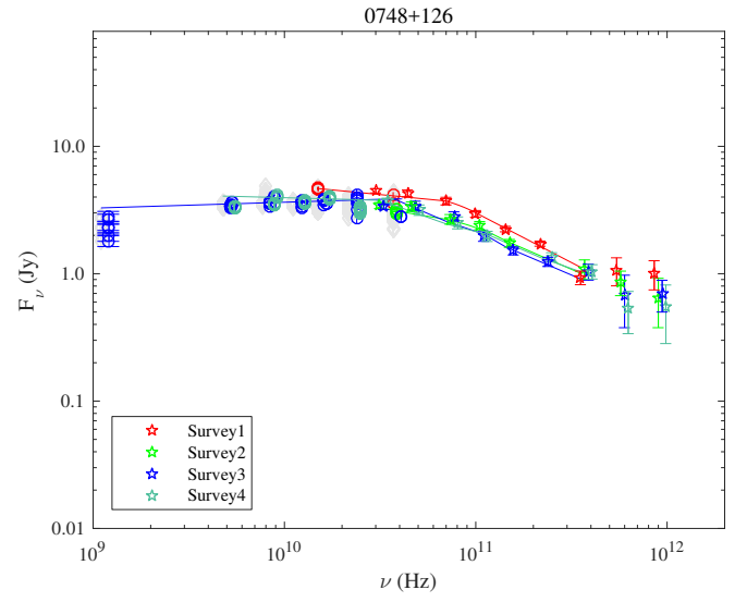
Fig. 1.34. 0748+126.
