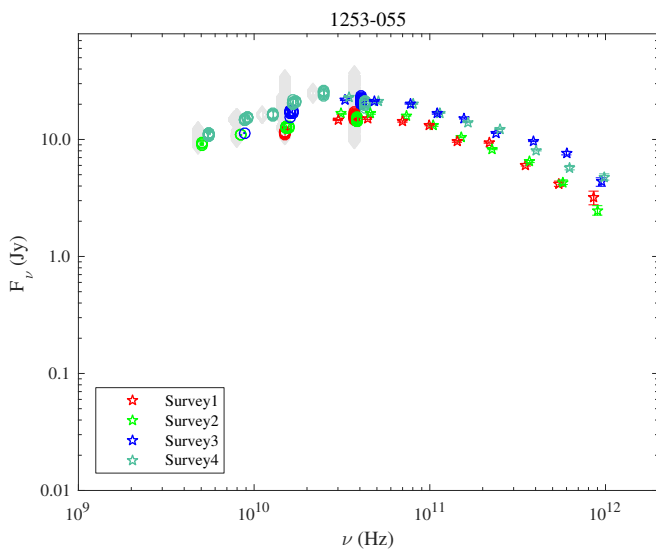
Fig. 1.59. 1253-055.
