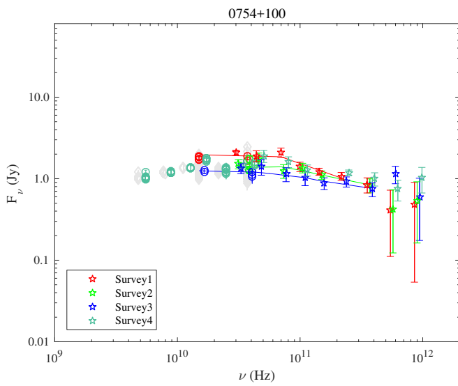
Fig. 1.35. 0754+100.
