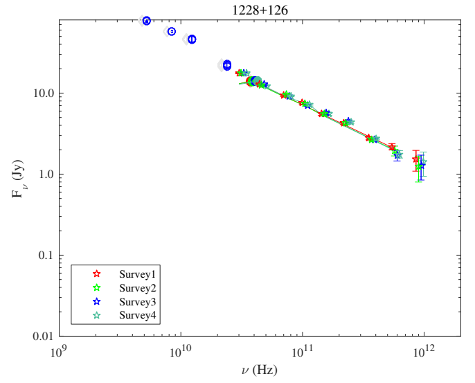
Fig. 1.58. 1228+126.
