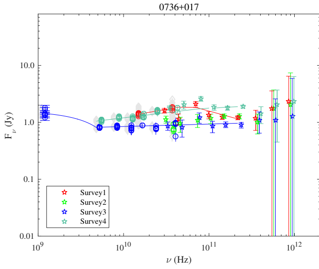
Fig. 1.33. 0736+017.
