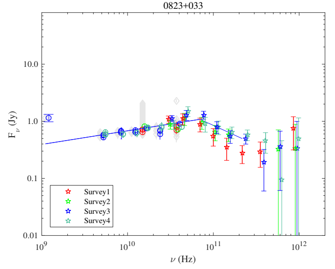
Fig. 1.38. 0823+033.
