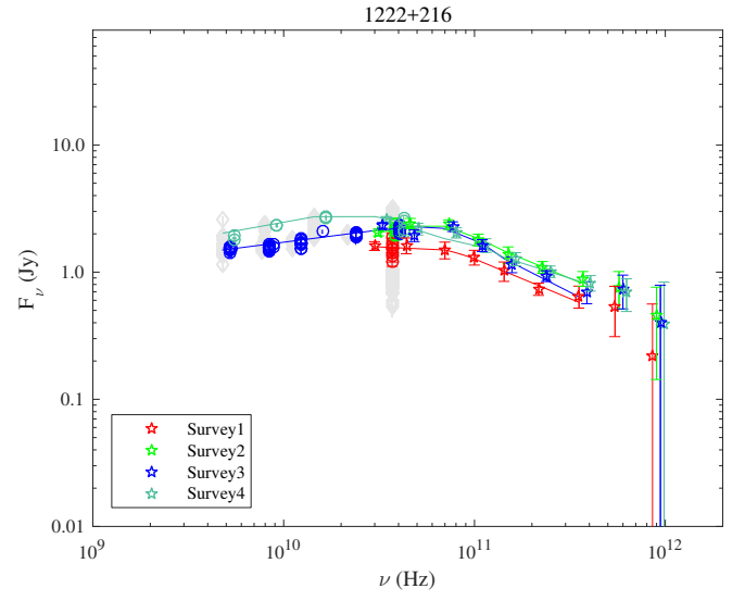
Fig. 1.56. 1222+216.
