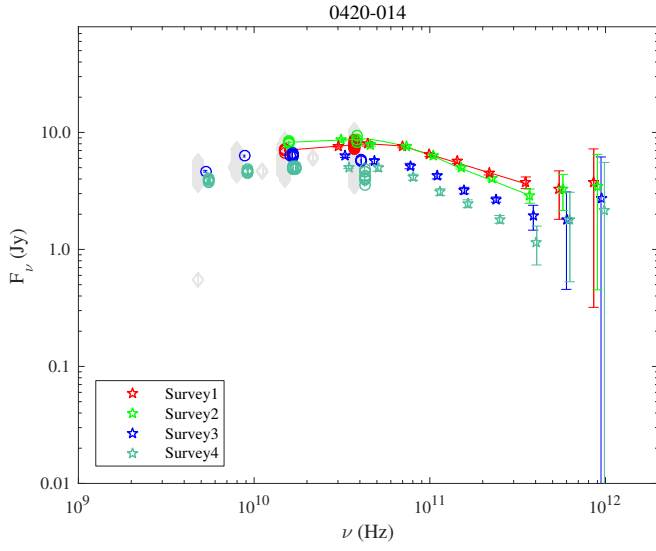
Fig. 1.21. 0420-014.
