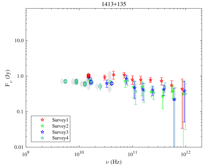
Fig. 1.62. 1413+135.
