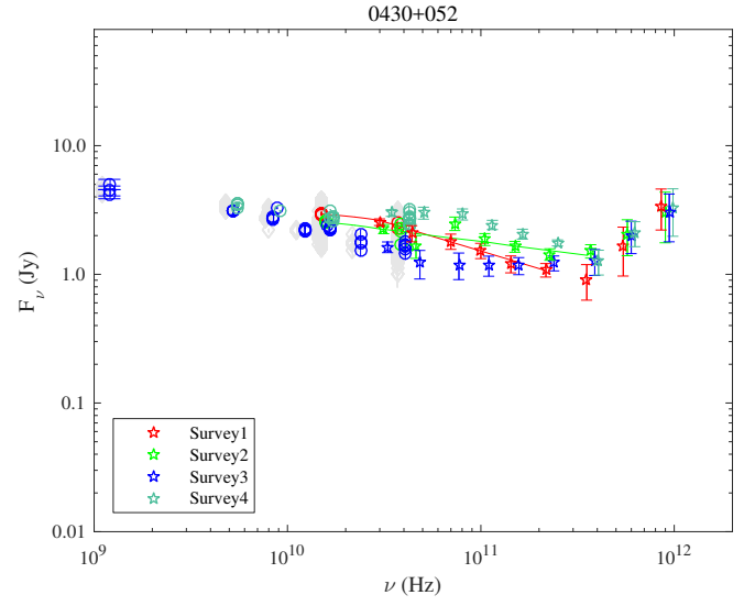
Fig. 1.22. 0430+052.
