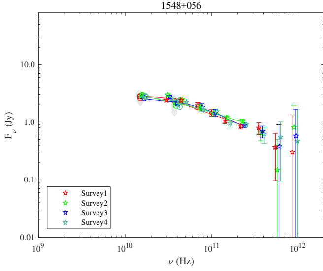
Fig. 1.67. 1548+056.
