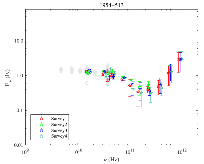
Fig. 1.84. 1954+513.
