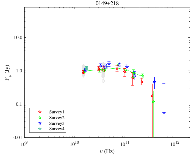
Fig. 1.8. 0149+218.
