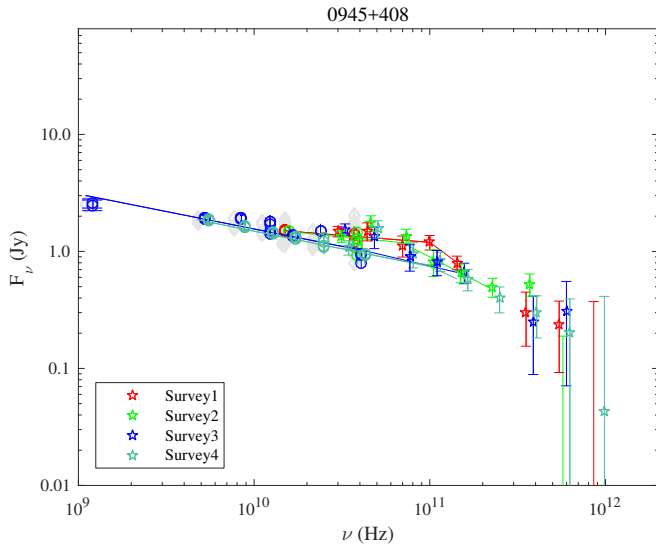
Fig. 1.45. 0945+408.
