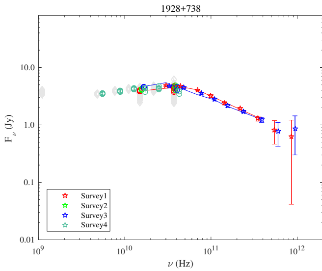
Fig. 1.83. 1928+738.
