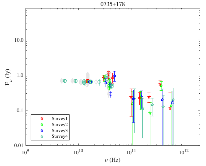
Fig. 1.32. 0735+178.
