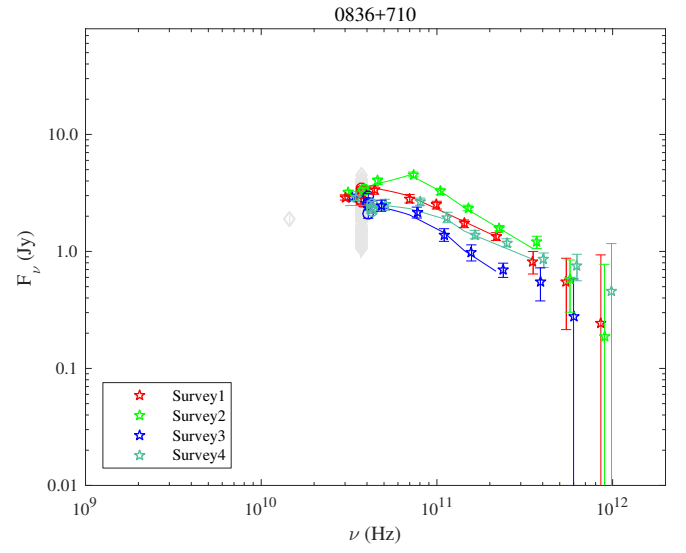
Fig. 1.40. 0836+710.
