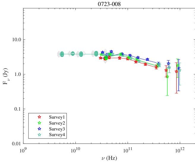
Fig. 1.31. 0723–008.
