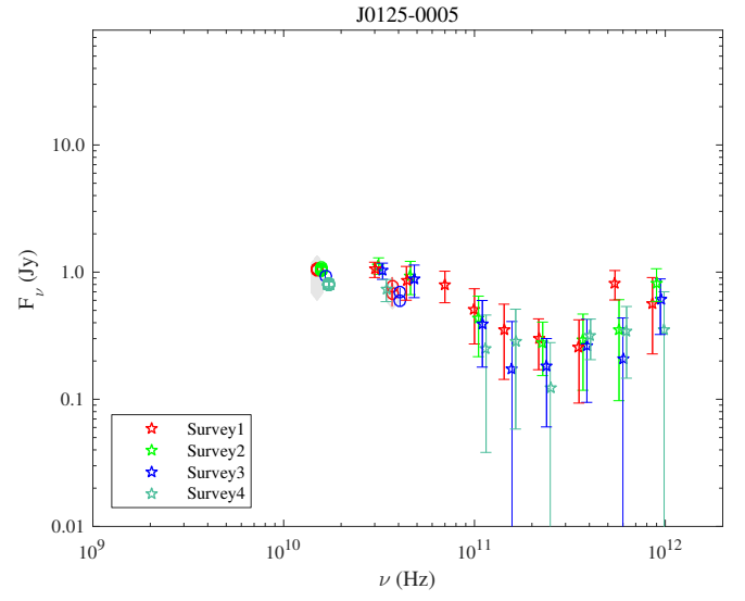
Fig. 1.6. J0125-0005.
