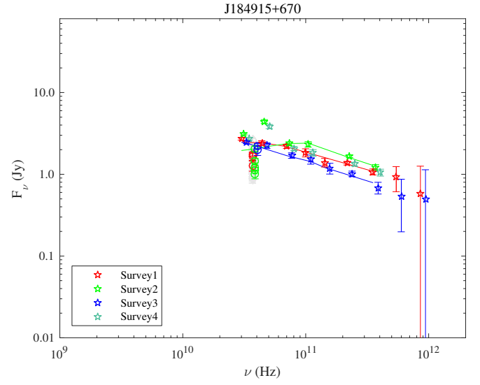
Fig. 1.82. J184915+670.
