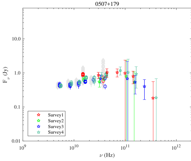
Fig. 1.25. 0507+179.
