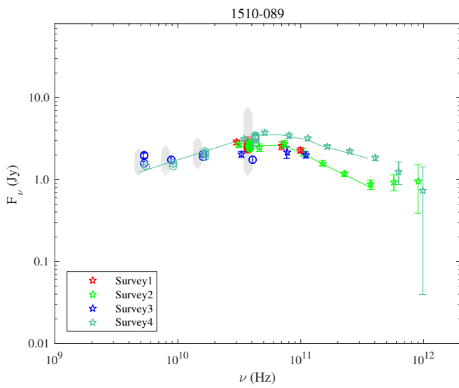
Fig. 1.65. 1510-089.
