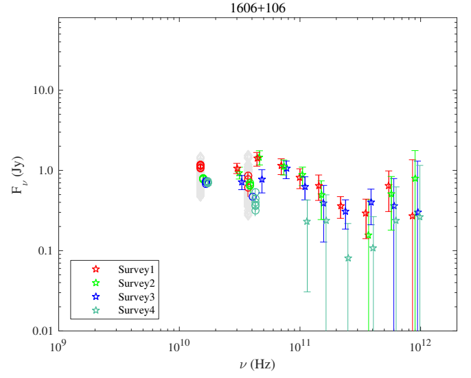
Fig. 1.68. 1606+106.
