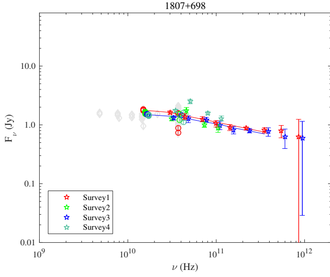
Fig. 1.79. 1807+698.
