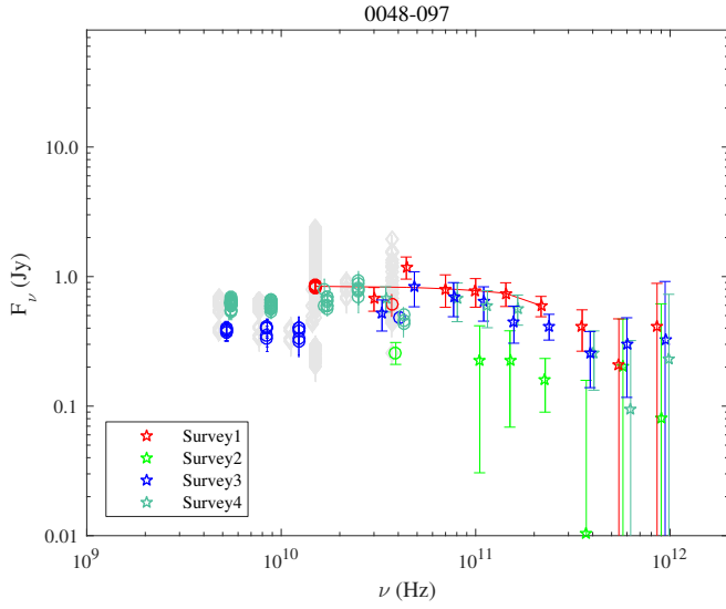
Fig. 1.3. 0048-097.
