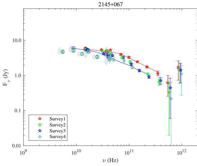
Fig. 1.93. 2145+067.
