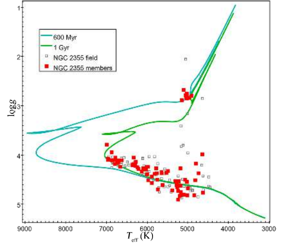
Fig. B.183. Kiel diagram for NGC 2355.
