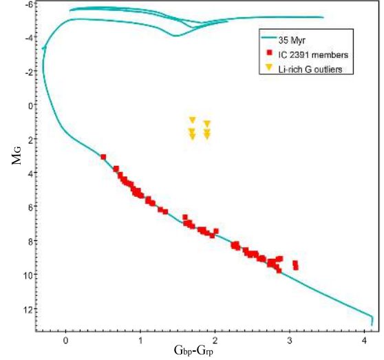
Fig. B.66. CMD for IC 2391.
