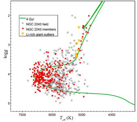
Fig. B.231. Kiel diagram for NGC 2243.
