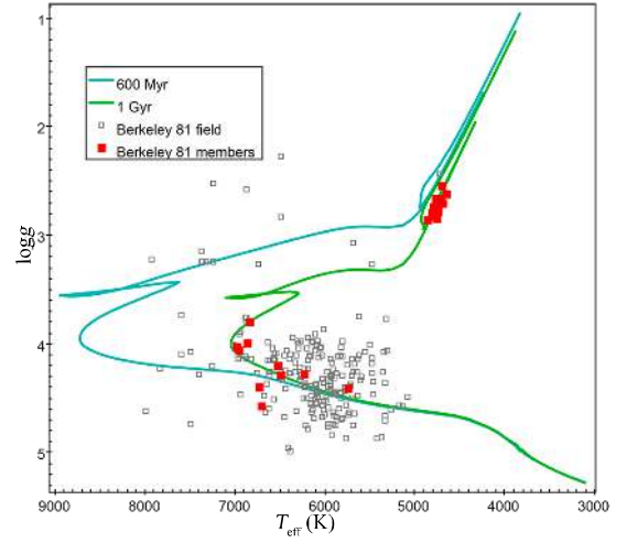
Fig. B.177. Kiel diagram for Berkeley 81.
