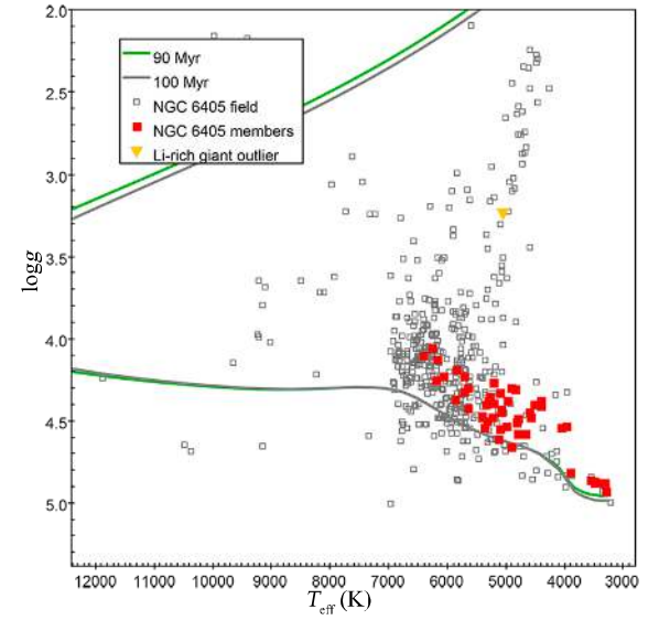
Fig. B.89. Kiel diagram for NGC 6405.
