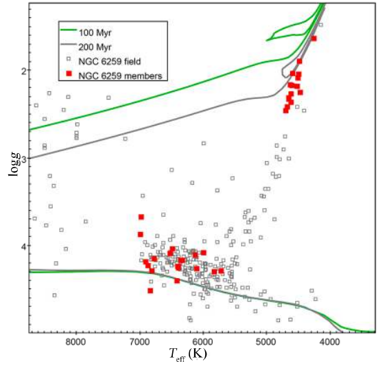
Fig. B.123. Kiel diagram for NGC 6259.
