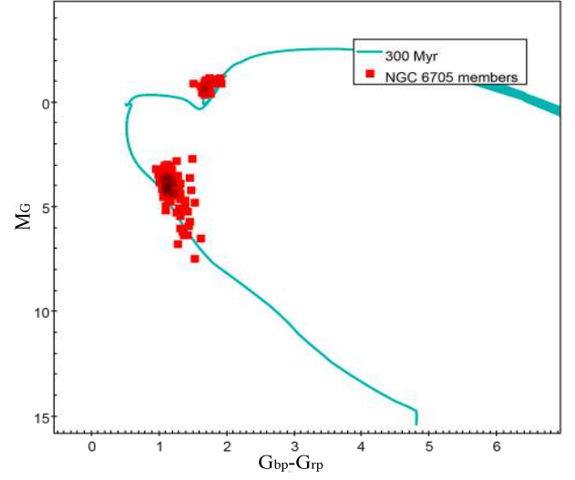
Fig. B.128. CMD for NGC 6705.
