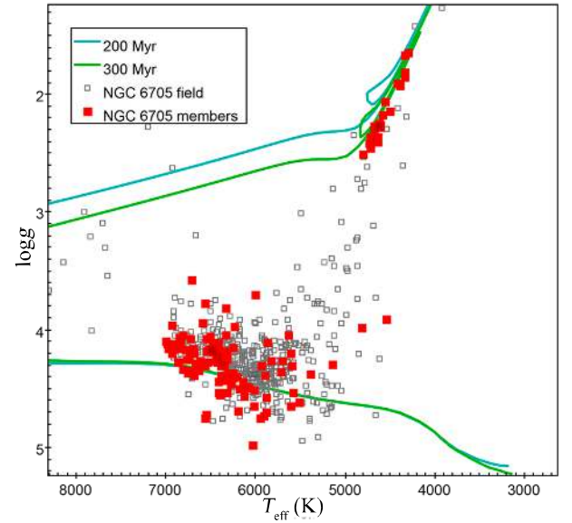
Fig. B.129. Kiel diagram for NGC 6705.
