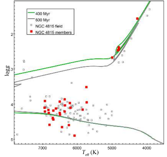
Fig. B.153. Kiel diagram for NGC 4815.
