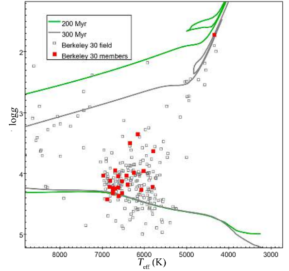
Fig. B.135. Kiel diagram for Berkeley 30.
