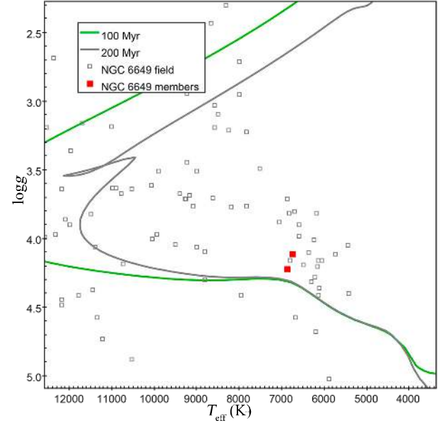
Fig. B.105. Kiel diagram for NGC 6649.
