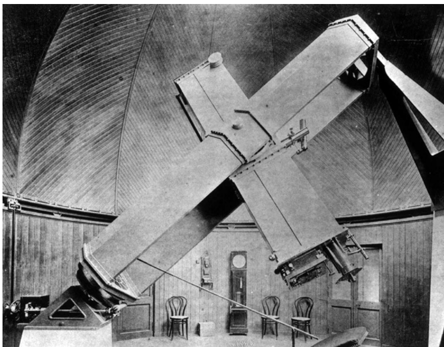
L'astrografo Henry-Gautier, il doppio telescopio visuale e fotografico, utilizzato per la fotografia del cielo (1891).
