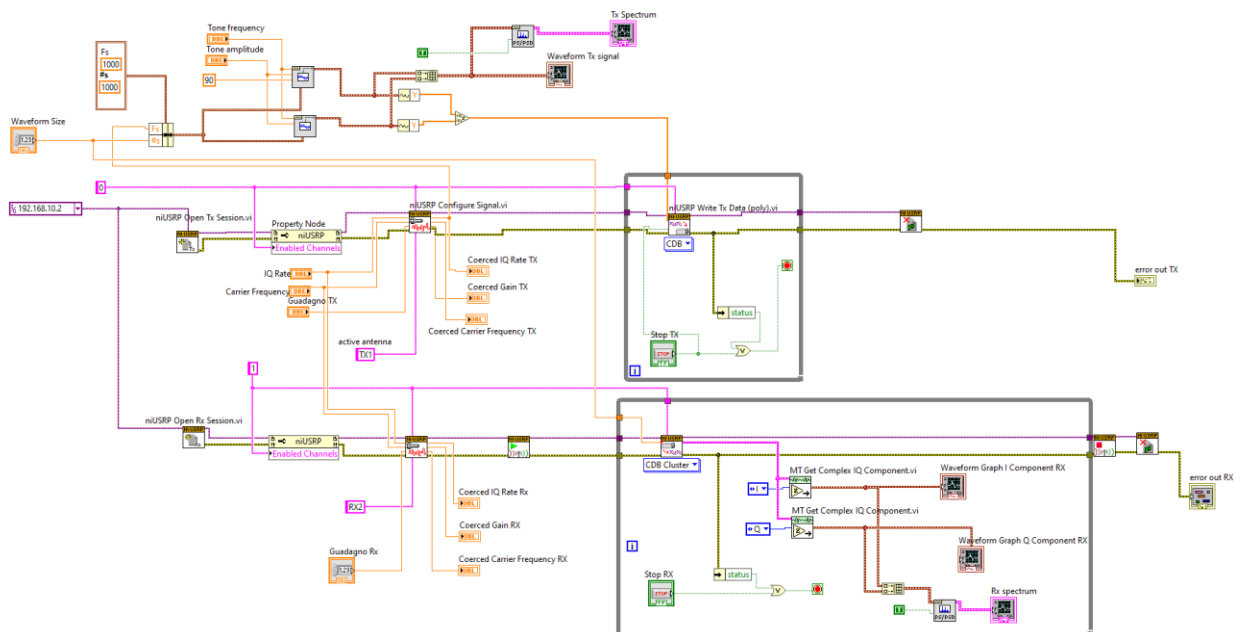
Figura 8: Prototipo in banda C. Schema a blocchi LABVIEW.
