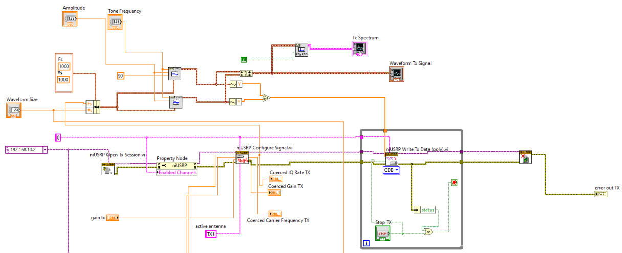
Figura 12.a: schema a blocchi LABVIEW del trasmettitore.
