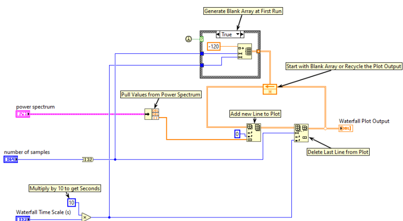
Figura 13: Schema a blocchi LABVIEW del VI “generate waterfall plot”.
