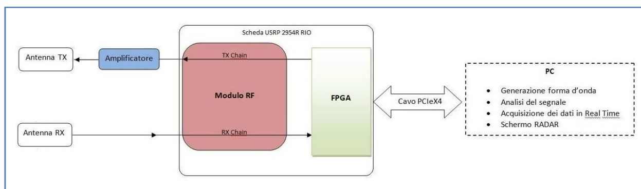
Figura 6: schema dell'unità RADAR realizzata mediante la scheda USRP-2954R.
