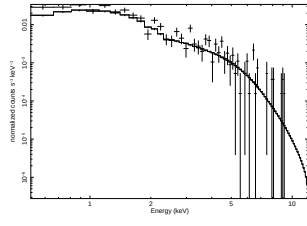
3XLSS J021606.0-051720
