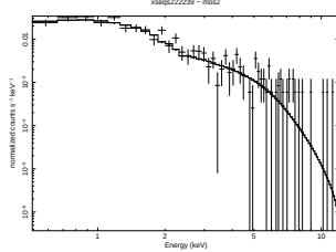
3XLSS J020423.1-040851
