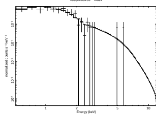
3XLSS J020559.6-063736
