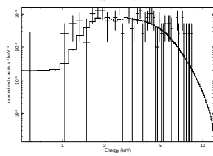
3XLS J022143.9-053146
