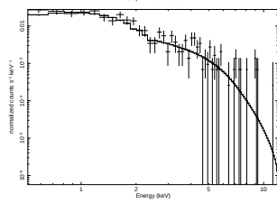
3XLSS J020534.0-073705
