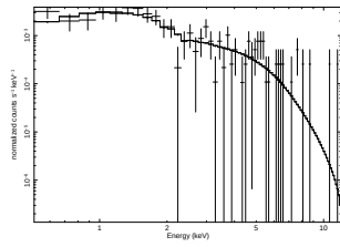
3XLS J022258.0-041840
