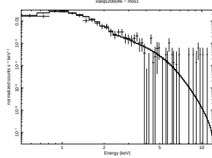
3XLS J022012.0-034111
