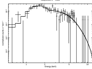
3XLSS J023040.6-040752
