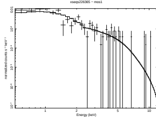
3XLSS J023304.3-053946 1
