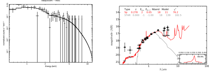
3XLSS J020207.0-055858
