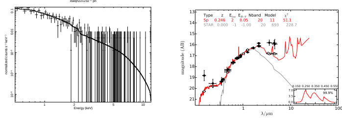
3XLSS J023322.1-045505
