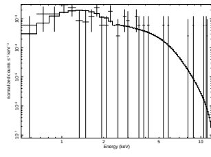
3XLS J021329.1-053909
