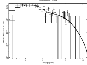
3XLS J023440.2-050231
