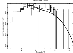
3XLSS J022541.3-032624
