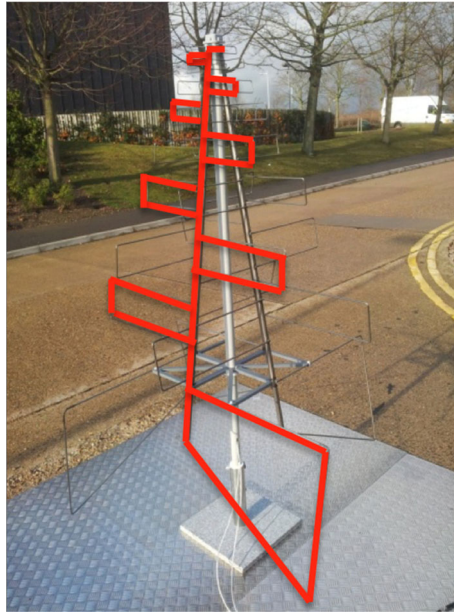
Fig. 2 SKALA-1. 1 arm highlighted in red
