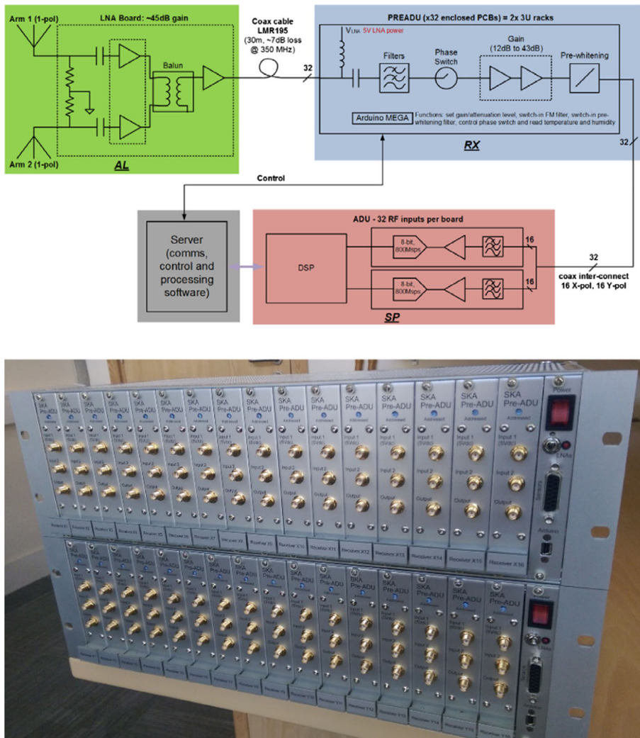
Fig. 6 AAVS0 RF system
