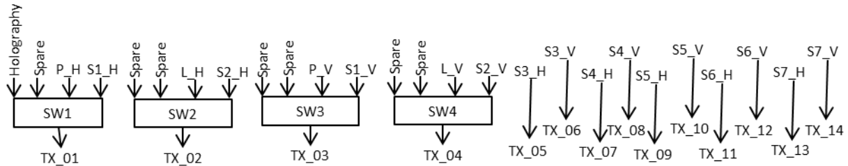
Fig. 8.8 Collegamenti della PFR Switch matrix
