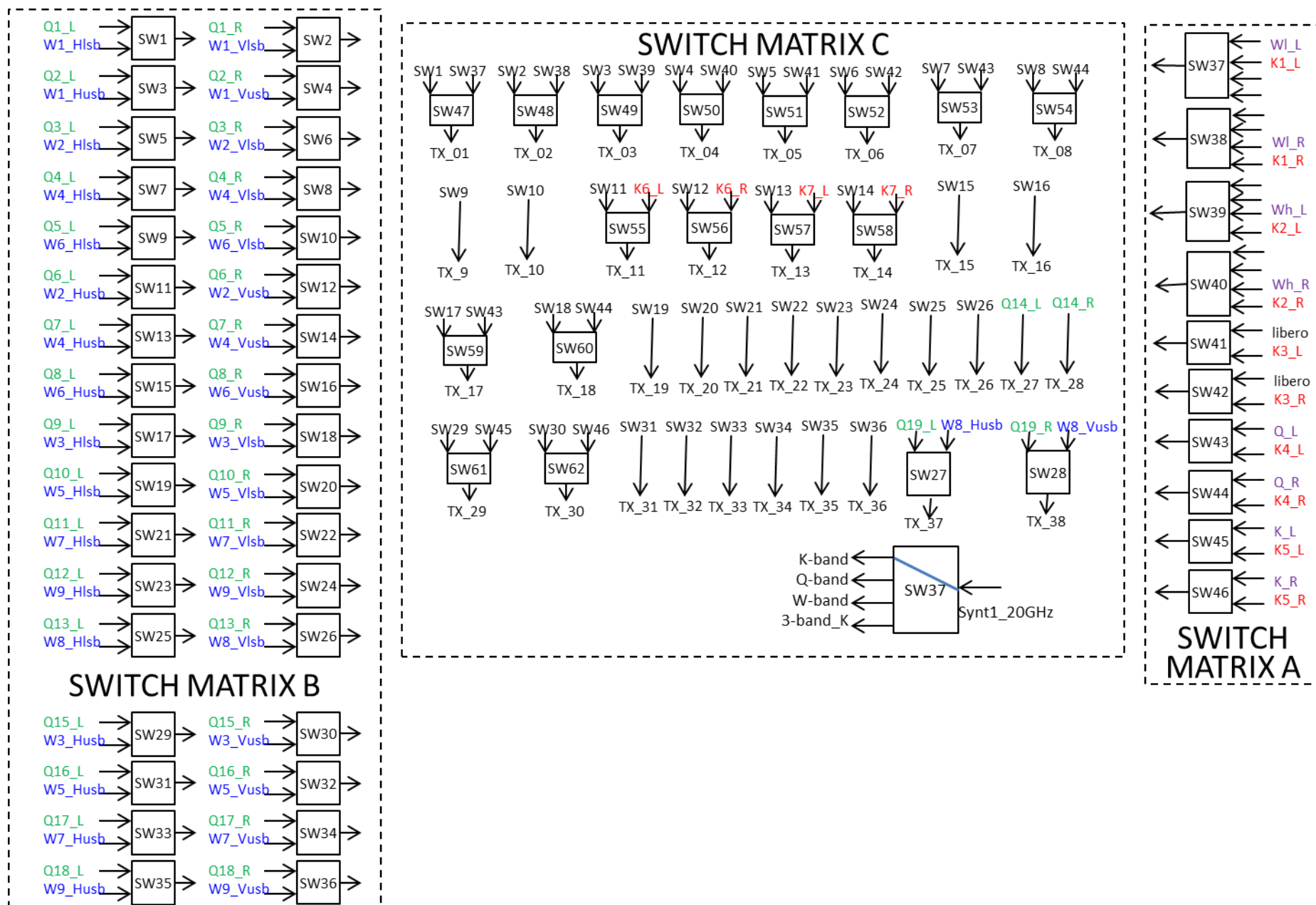
Fig. 8.7 Schema dei collegamenti per la soluzione "a bus". Q-band colore verde; W-band colore blu; K-band colore rosso; 3-band colore viola.
