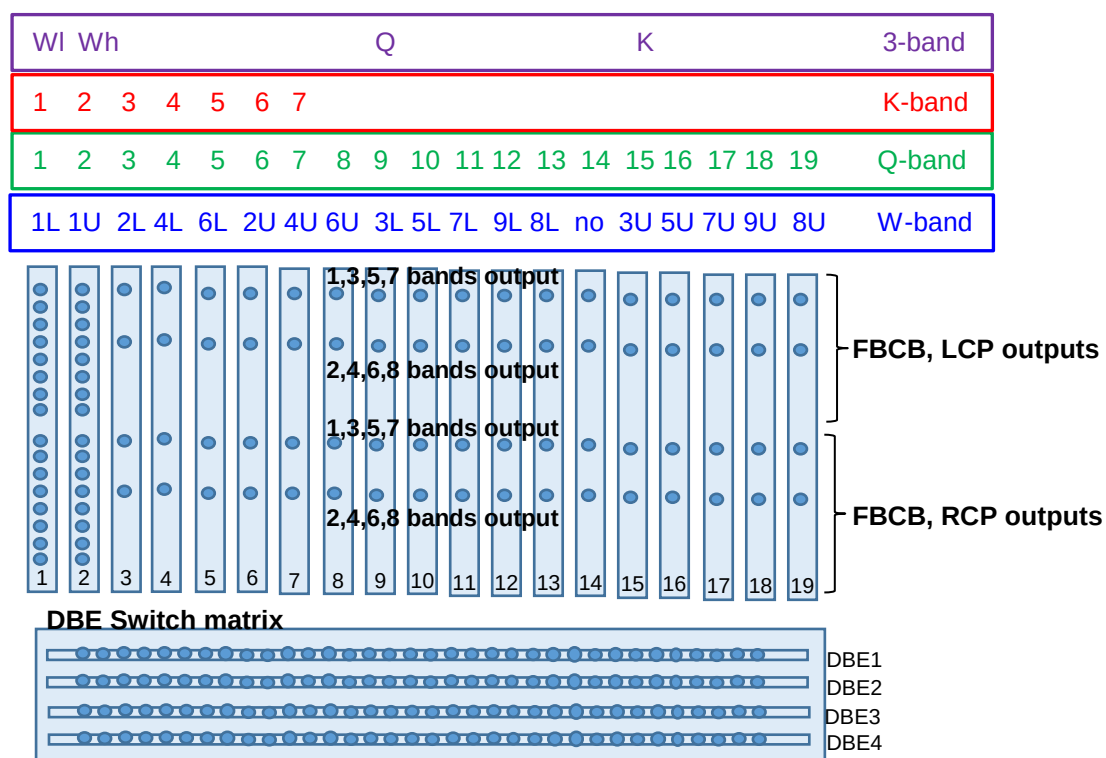
Fig. 8.10 Sistema FBCB con DBE switch matrix
