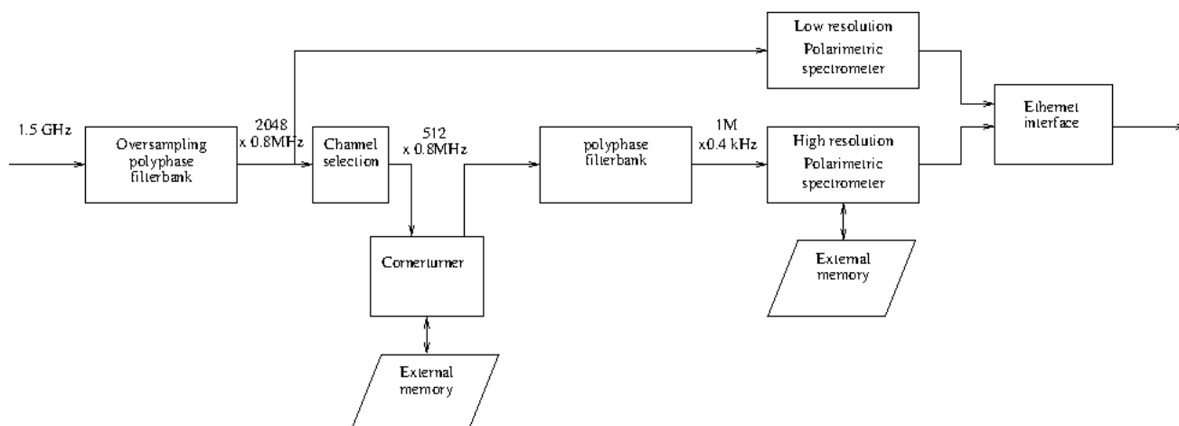
Fig. 3.3 Struttura di massima di spettrometro ad altissima risoluzione
