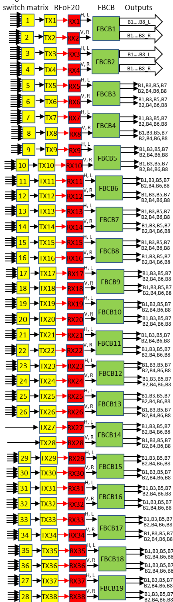
Fig. 9.3 Instradamento delle uscite ricevitori alle matrici di commutazione e le uscite di queste ai BEnds
