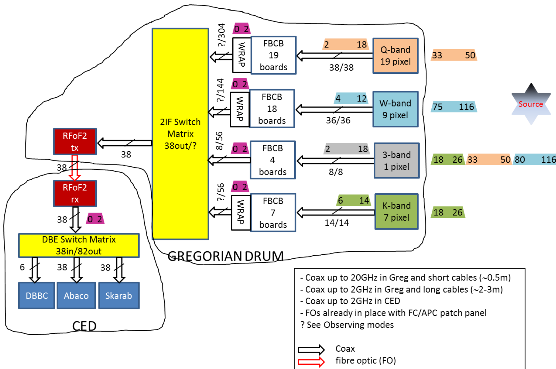
Fig. 5.2.1 Diagramma a blocchi della soluzione B: uso di link ottici banda stretta 2GHz e sistemi FBCB separati
