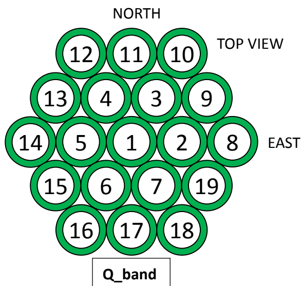
Fig. 8.1a 19-feed Q-band
