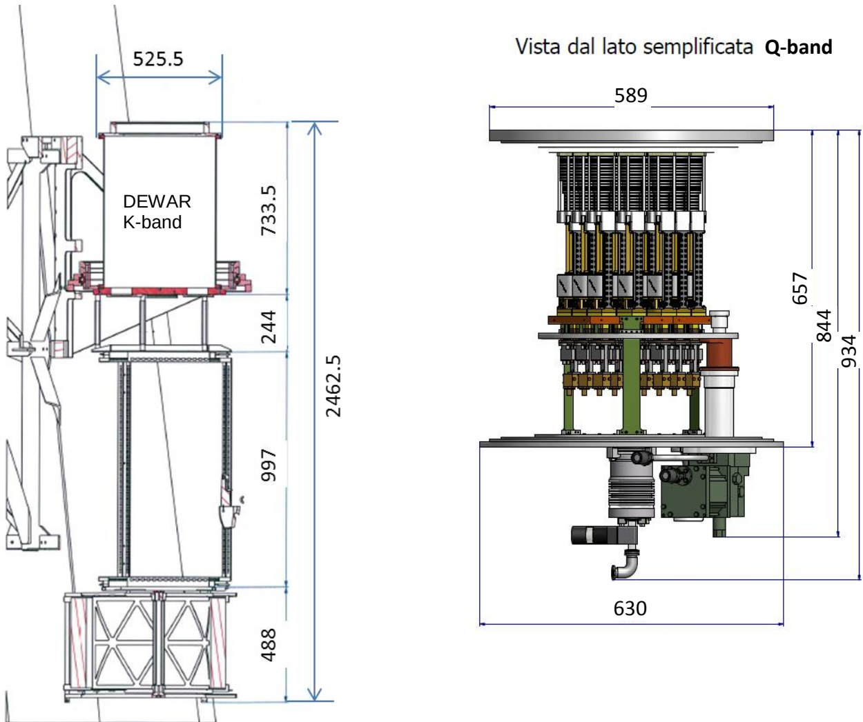
Fig. 6.1 (sinistra) Dimensioni essenziali del multifeed K-band presente sul tamburo gregoriano di SRT e confronto col dewar Q-band (destra)
