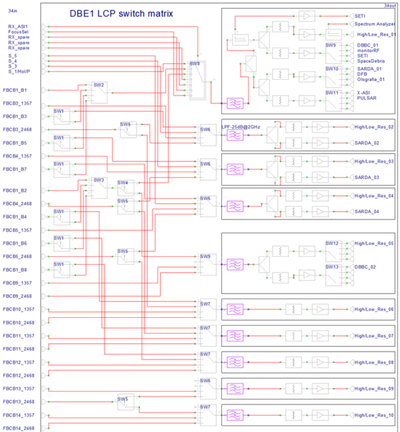
Fig. 8.11 Schematico della scheda 1 del DBE switch matrix per utenze LCP o H. Sul lato sinistro arrivano le uscite delle schede FBCB, sul lato destro partono le connessioni ai vari back-end.
