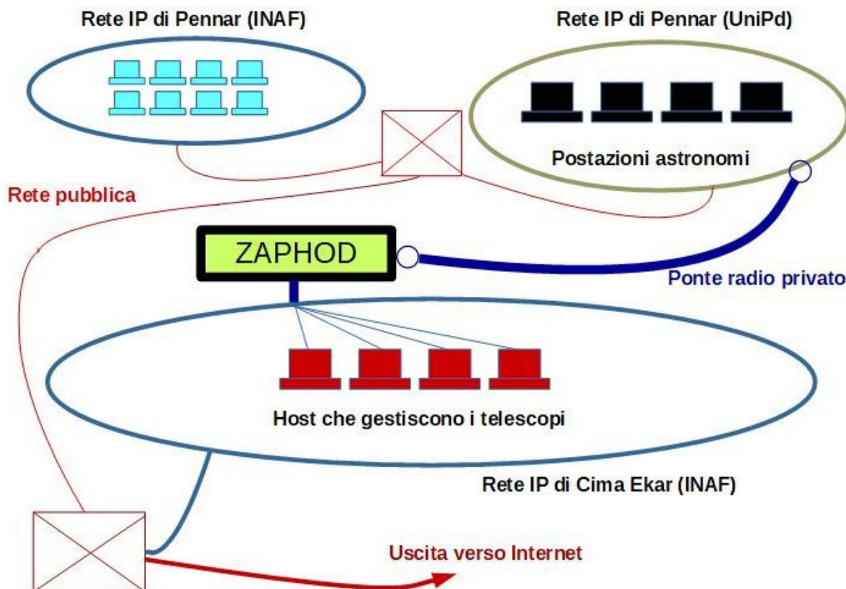
Figura 1 – Schema di base delle reti di Asiago
