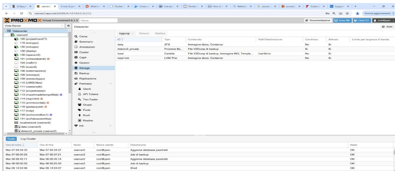
Figura 1 - Schermata Principale
