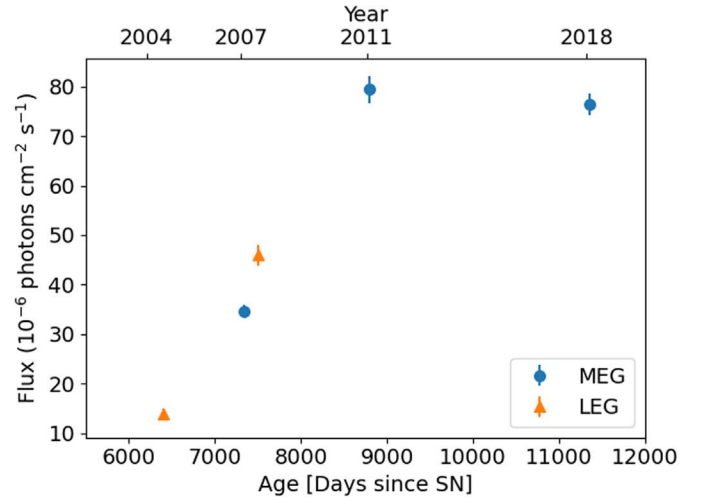
(b) Si (He \alpha )
