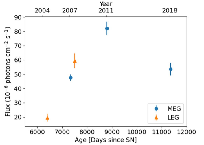
(d) Mg (He \alpha )
