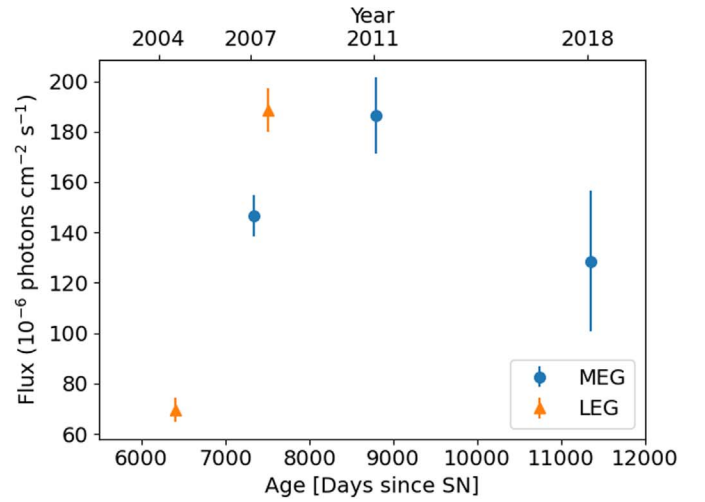
(f) Ne (He \alpha )
