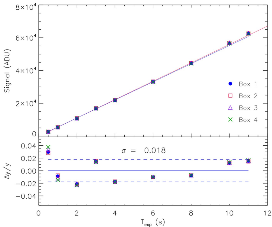
Fig. 4. ( In alto ) Segnale medio in ADU in funzione del tempo di posa per le 4 aree di 1 \text{ mm}^2 di Fig. 2 (simboli come nella legenda). Il best-fit lineare ai dati è rappresentato dalla linea rossa. La relazione lineare C=A \cdot T_{exp} è visualizzata con la linea blu. ( In basso ) Differenza dei valori rispetto al best-fit . La deviazione standard è \sigma=1.8 \% .
