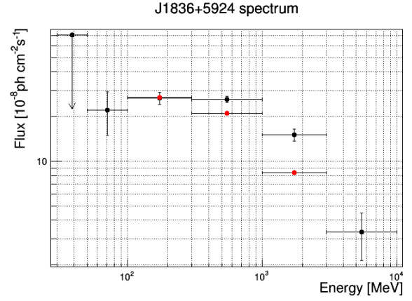
(d) 2AGL J1836+5924 (PSR J1836+5925)
