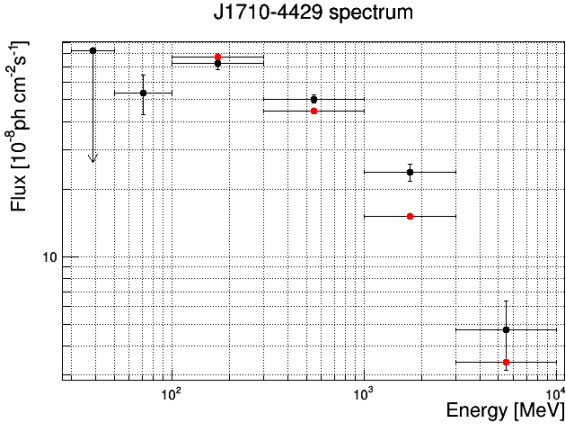
(c) 2AGL J1710-4429
