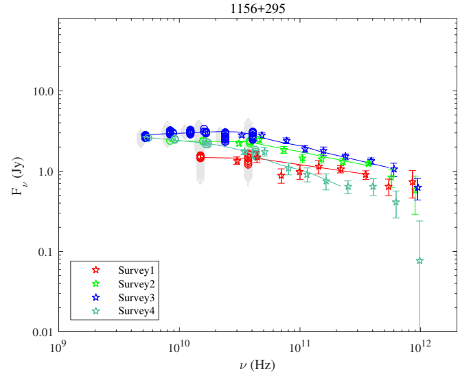
Fig. A.54. 1156+295.
