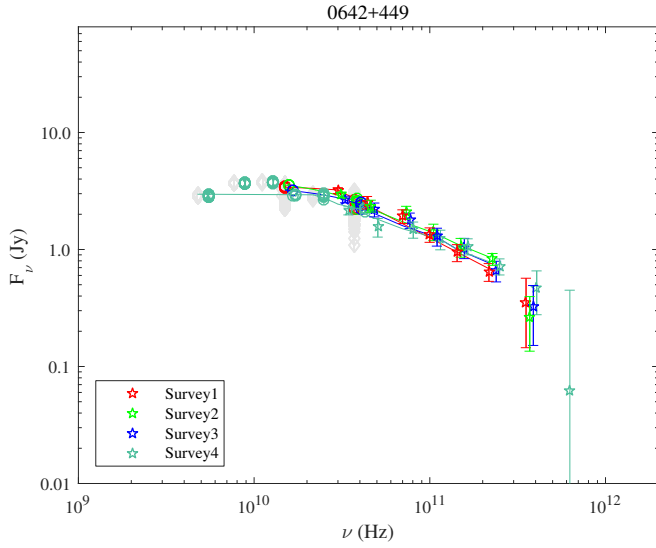
Fig. A.29. 0642+449.
