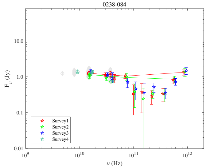
Fig. A.14. 0238-084.
