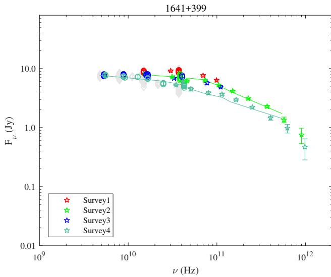
Fig. A.73. 1641+399.
