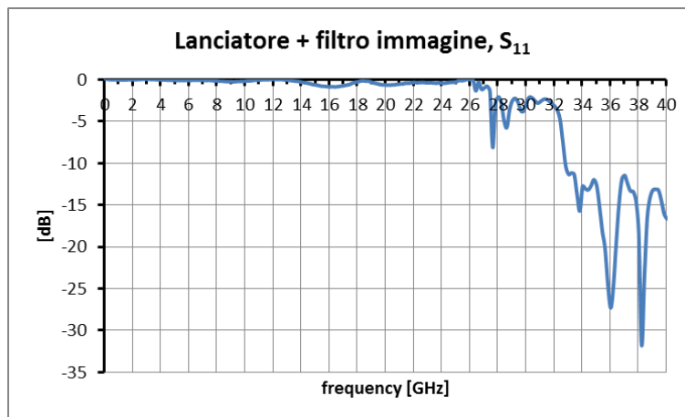
Fig. 4.12 Parametro S_{11} dello stadio d'ingresso del Q-CONV
