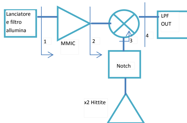
Fig. 4.4 Schema a blocchi
