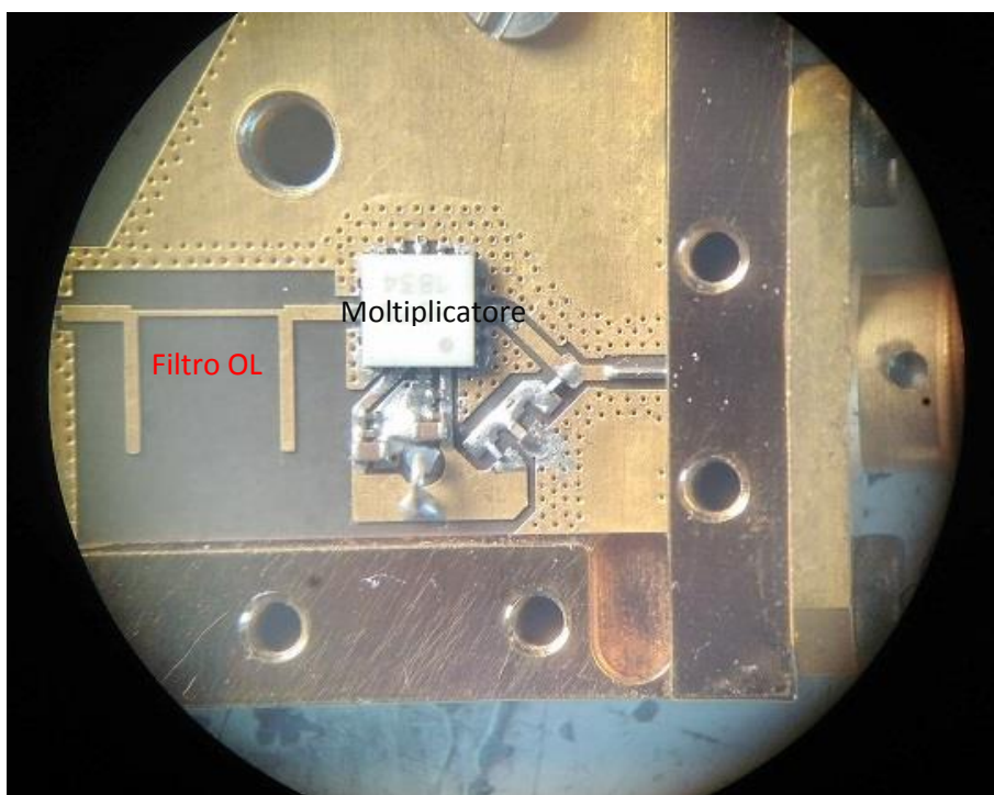
Fig. 3.16 Il moltiplicatore, quadrato bianco, e il filtro OL a sinistra
