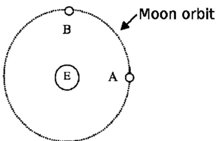
FIG. 11. Moon orbit.
