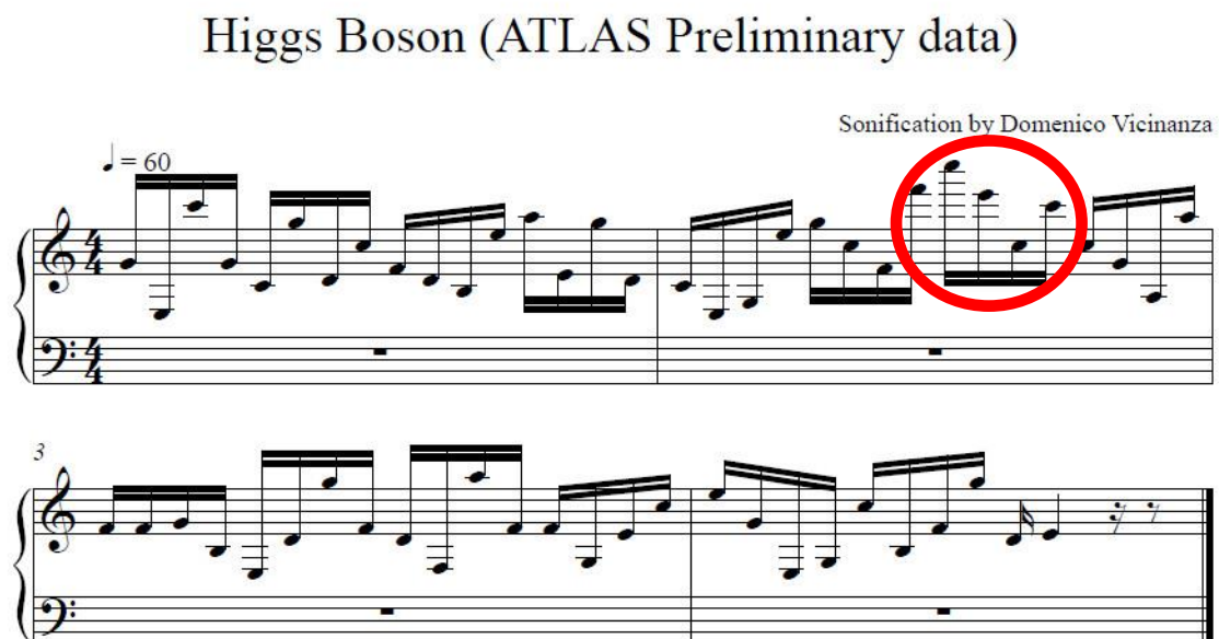
Figura 22 Sonificazione dei dati dell'esperimento che ha portato alla rivelazione del Bosone di Higgs.
