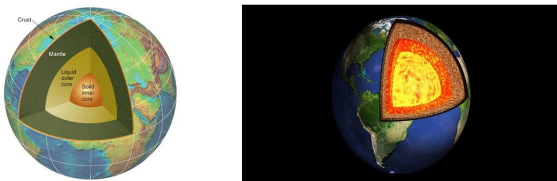
Figura 13 Schematizzazione 76 (a sinistra) e artist impression 77 (a destra) della conformazione interna della Terra.
