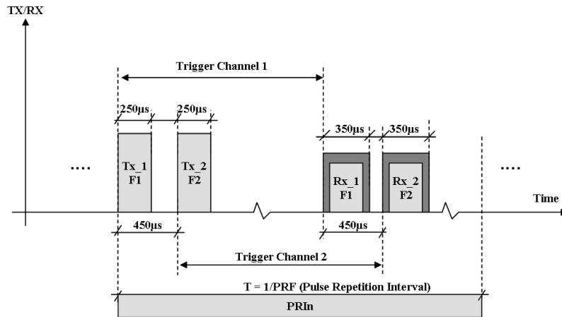
Fig. 2.3 PRI Timings
