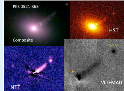
Fig. 1 Multiband images of PKS 0521-365
