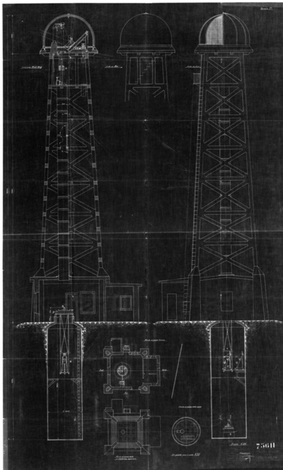
Fig. 15 – Blueprints della Torre Solare, Officine Galileo, 6 dicembre 1920. [Archivio Storico INAF – Osservatorio Astrofisico di Arcetri]
