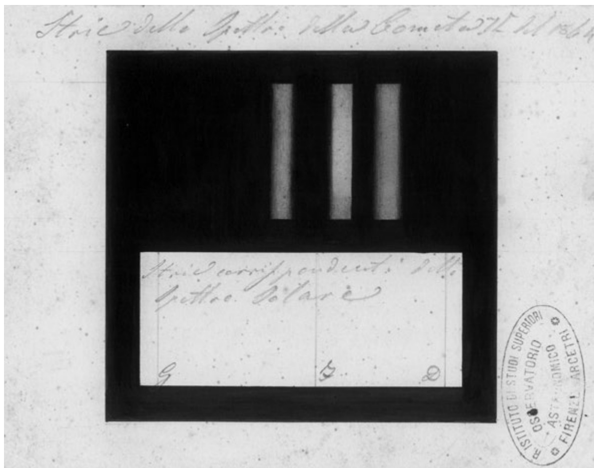
Fig. 7 – Lo spettro della cometa C/1864 N1. [Archivio Storico INAF – Osservatorio Astrofisico di Arcetri]
