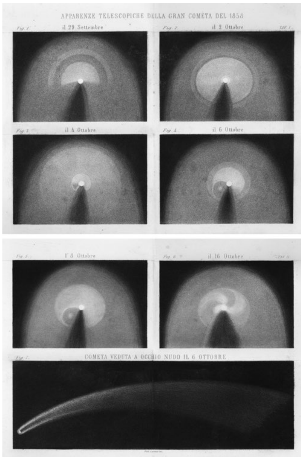
Fig. 3 – La cometa C/1858 LI. [da Annuario dell'I. e R. Museo di Fisica e Storia Naturale per il 1859 , Le Monnier, Firenze 1858]
