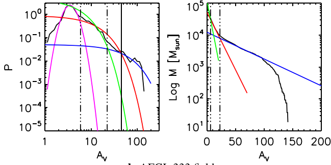
b AFGL 333 field
