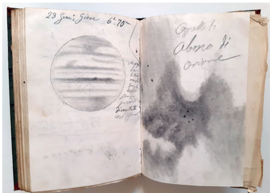
FIG. 3.9. Drawing of Jupiter dated 23 January 1859 ( Osservazioni all'Equatoriale dal 23 giugno 1858 al 24 febbraio 1859 , INAF-Osservatorio Astronomico di Roma, Historical Archive, busta 43, n. 158)
