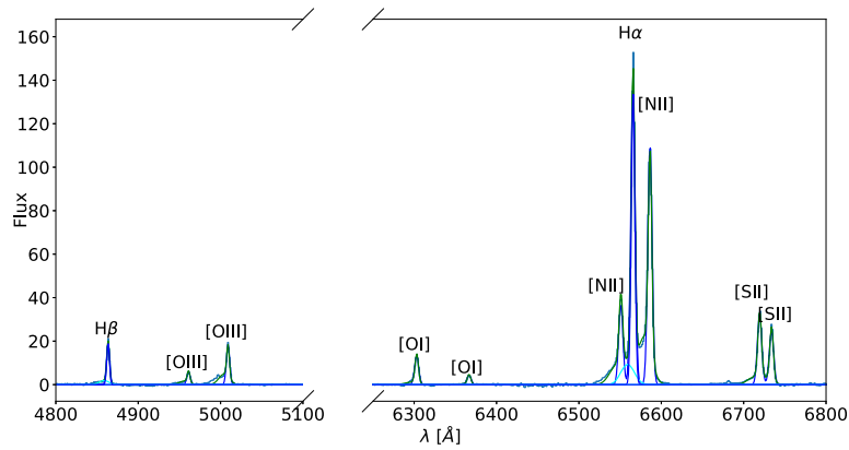
Figure D3. IRAS 14378–3651.
