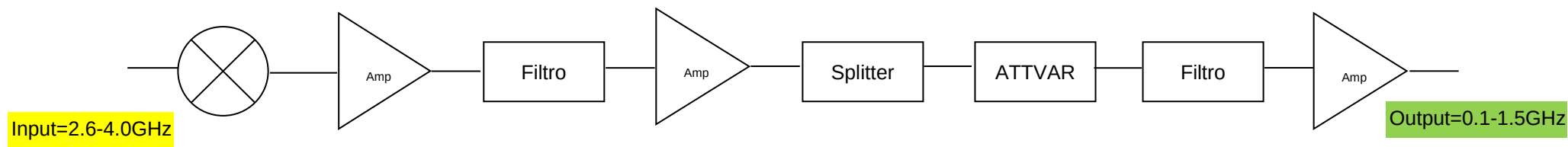
Fig. 1.4 2° Conversione. Una catena per ogni polarizzazione
