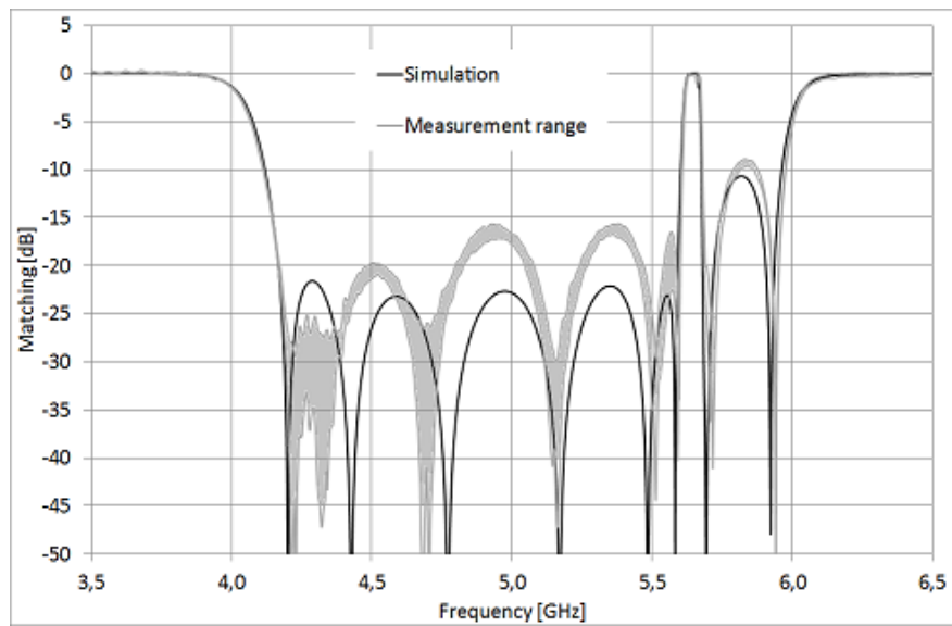
Fig. 3.5 Return loss dei tre filtri HTS prodotti
