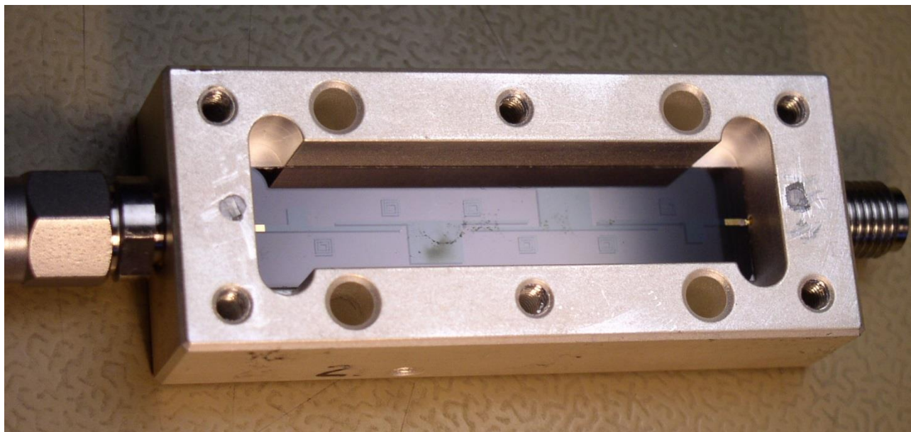
Fig. 3.1 Immagine del circuito del filtro HTS
