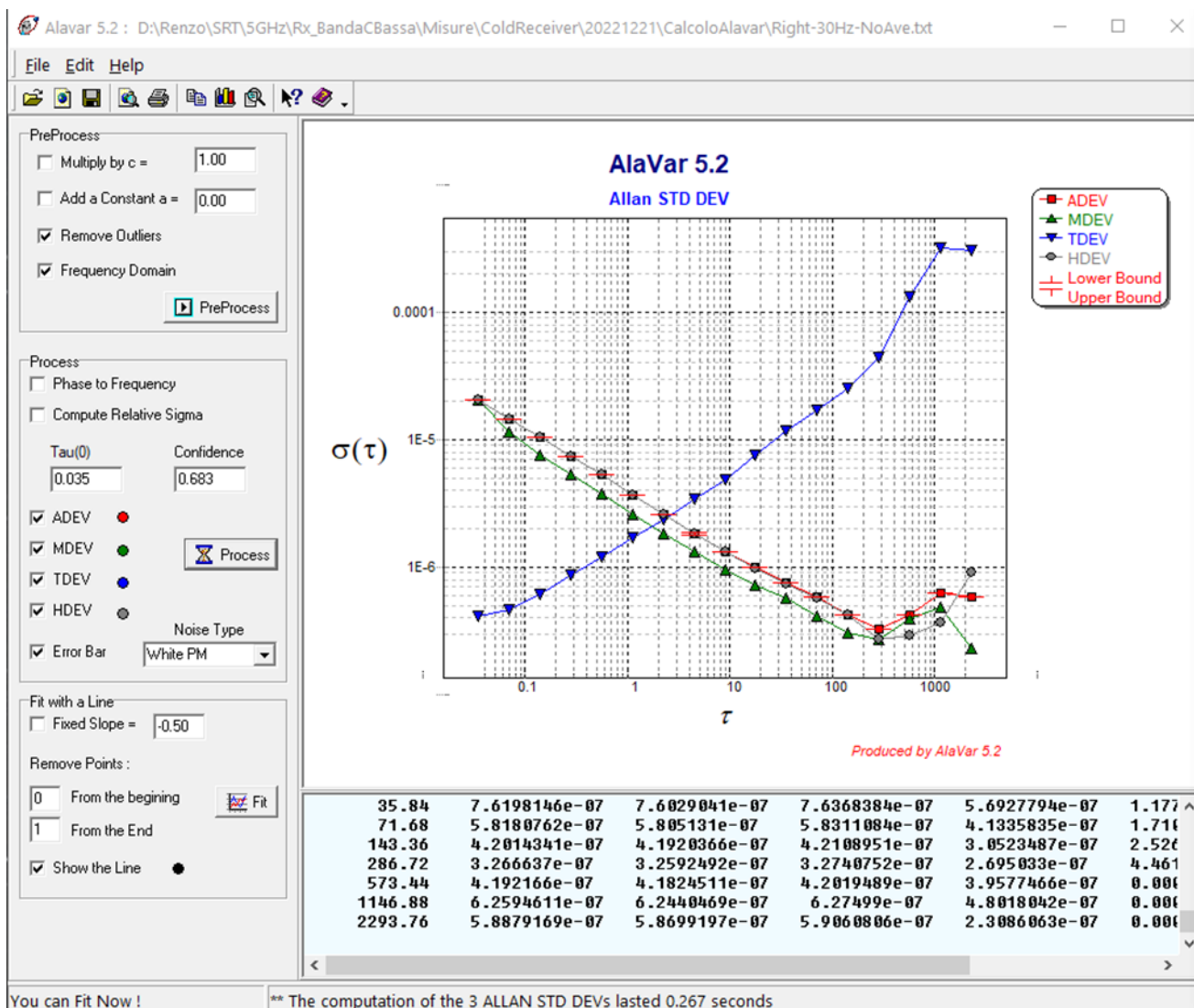
Fig. 10.4 Deviazione standard di Allan, RCP. Si consideri la curva rossa ADEV
