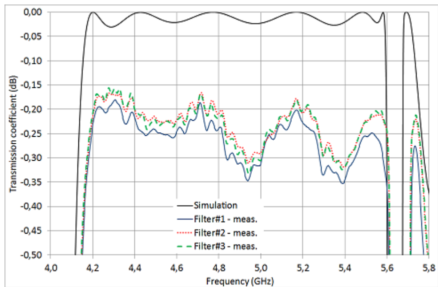
Fig. 3.4 Insertion loss dei tre filtri HTS prodotti
