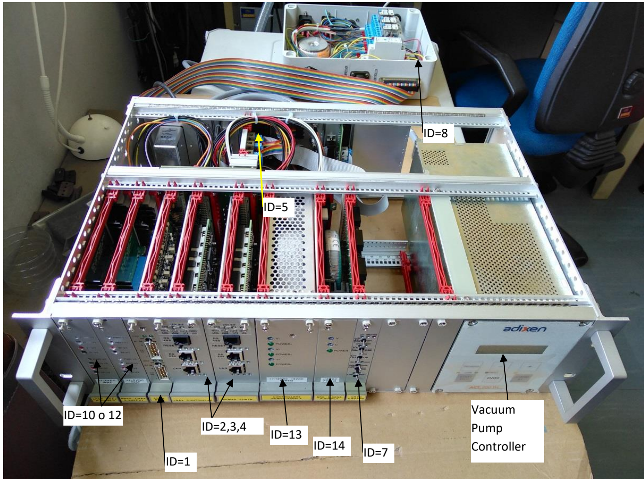
Fig. 5.1 Unità di M&C, vista di fronte
