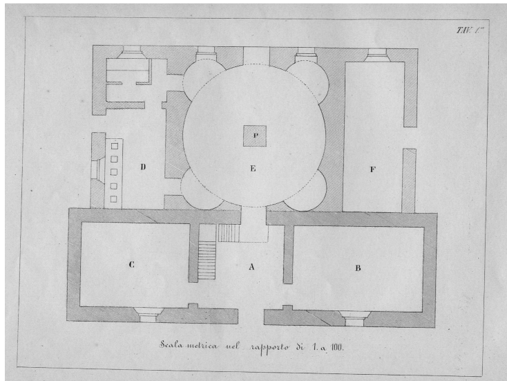
Fig. 7 – Pianta dell'Osservatorio Etneo, disegnata da Tacchini (da: Tacchini 1882)
