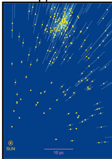
Hipparcos
