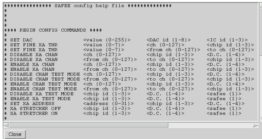
Figura 18 Finestra di help per i comandi testuali inseribili nel file di configurazione della SAFEE
