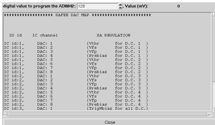
Figura 19 Finestra di help con la funzione di conversione tra il valore digitale dei DAC sulla SAFEE ed il valore analogico, e con la corrispondenza tra canali DAC di uscita degli integrati e polarizzazioni degli XA che vanno a regolare.
