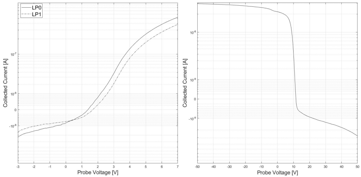
Figura 17 Caratteristiche I-V sonde di Langmuir (sinistra), caratteristica I-V sonda di Faraday (destra). Orientamento LP 0^\circ , Potenziale guard-ring -20V, configurazione sonda di Faraday collimata.
