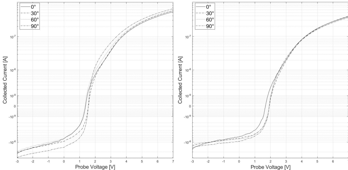
Figura 24 Effetto dell'orientamento delle LP rispetto al fascio: LP0 (sinistra), LP1 (destra)
