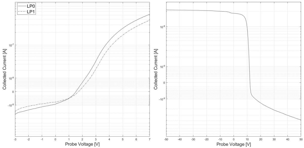
Figura 16 Caratteristiche I-V sonde di Langmuir (sinistra), caratteristica I-V sonda di Faraday (destra). Orientamento LP 0^\circ , Potenziale guard-ring -15V, configurazione sonda di Faraday collimata.
