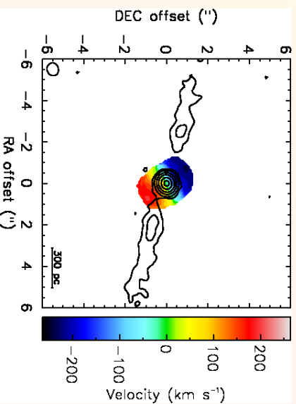
NGC 3557
