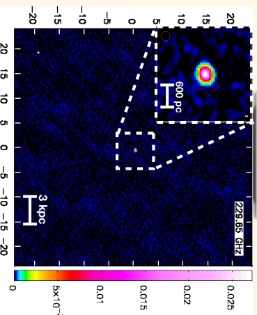
NGC 612
