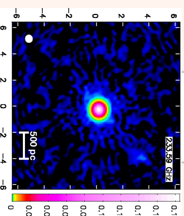
IC 4296
