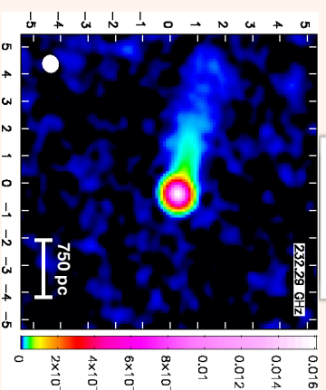
NGC 7075
