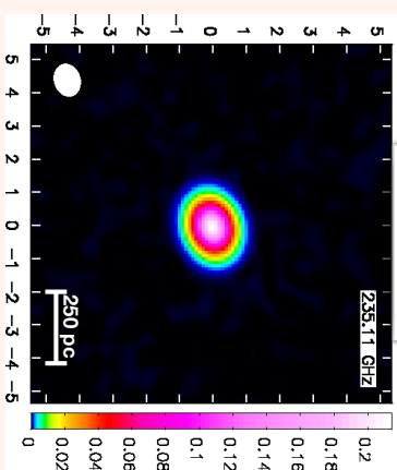
IC 1459
