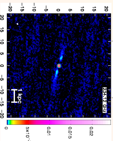
NGC 3557
