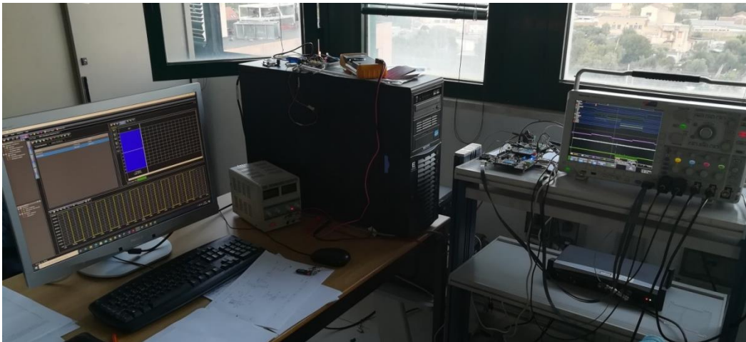
Figura 3. Banco di misura utilizzato per i test.
