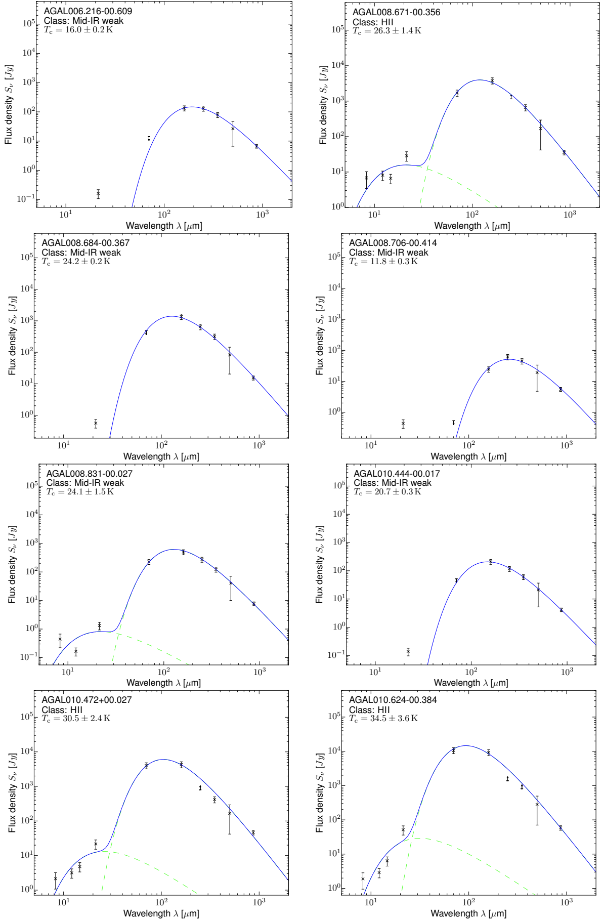
Fig. A.1. Source SEDs.
