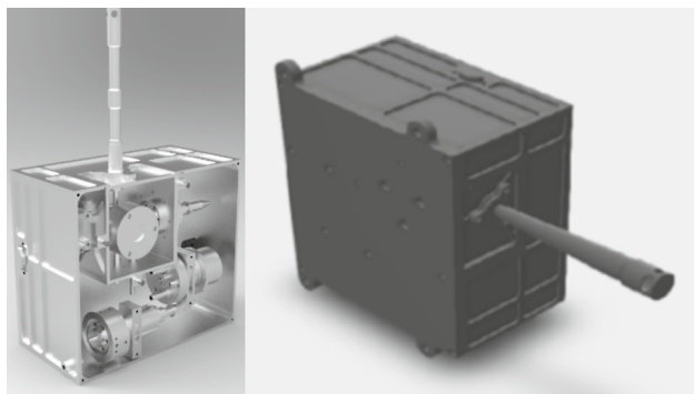
Fig. 1 MicroMED apparatus
