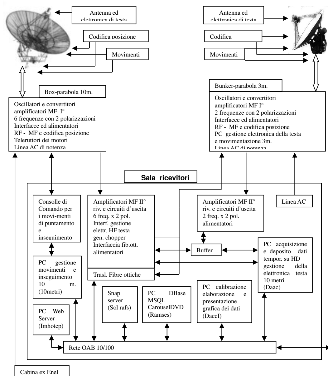
Figura 5 - Schema a blocchi / layout
