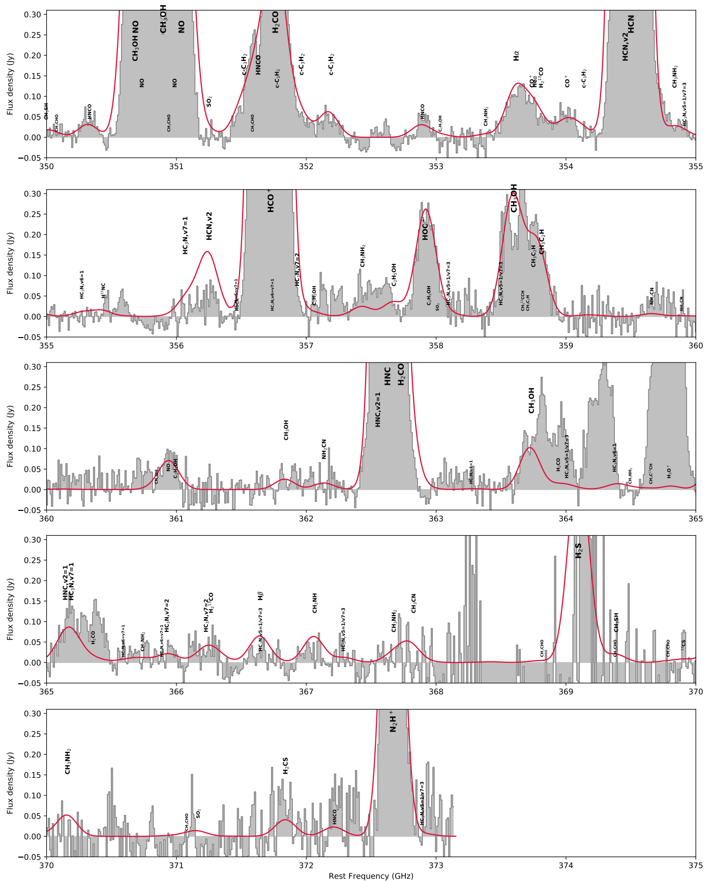
Fig. E.11. Same as Fig. E.2.
